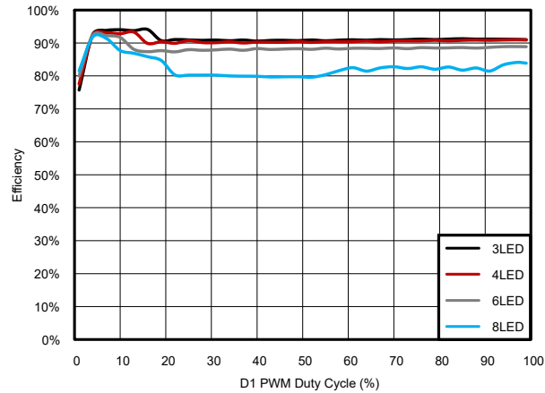
图 6-9. 7V 输入电压、0.5A 输出电流、20kHz PWM 下的 D1 效率
