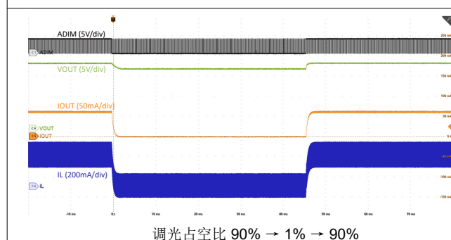
图 8-8. 调光瞬态
