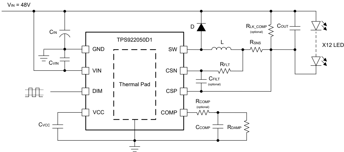
图 8-14. 48V 输入、1A 输出、12 片式 WLED、PWM 调光参考设计
