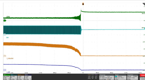
绿色：CSN，浅蓝色：SW，橙色：电感器电流，深蓝色：LED 电流
