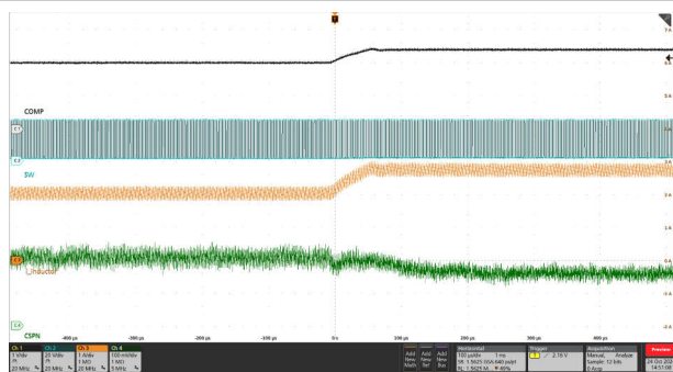
黑色：COMP，浅蓝色：SW，橙色：电感器电流，绿色：CSN
