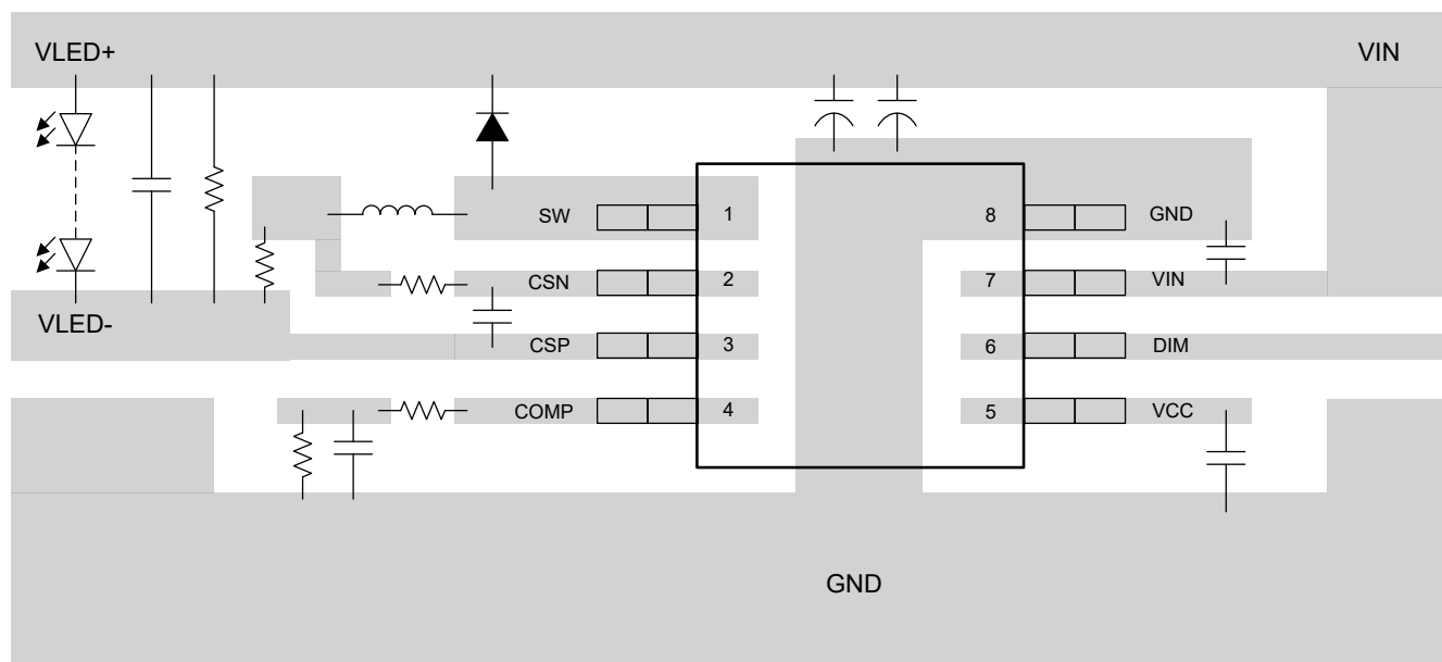
图 8-27. 8 引脚 SOT583 顶视图布局示例
