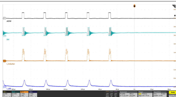
图 8-22. 在 DIM PWM = 100%、20kHz 时关断
