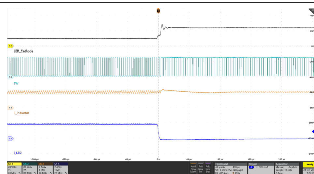
黑色：LED-，浅蓝色：SW，橙色：电感器电流，深蓝色：LED 电流
