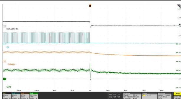
黑色：LED-，浅蓝色：SW，橙色：电感器电流，绿色：CSN
