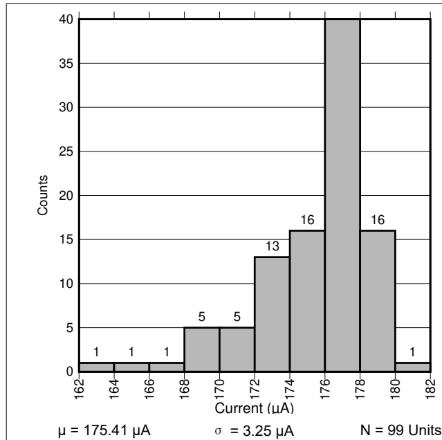
图 6-1. 8 MHz Oscillator Current
