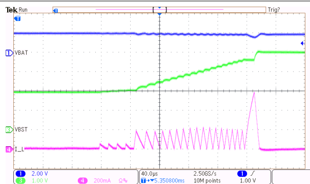
图 9-3. Boost Soft-Start
