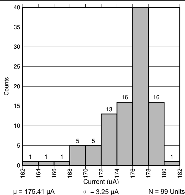
图 7-1. 8 MHz Oscillator Current
