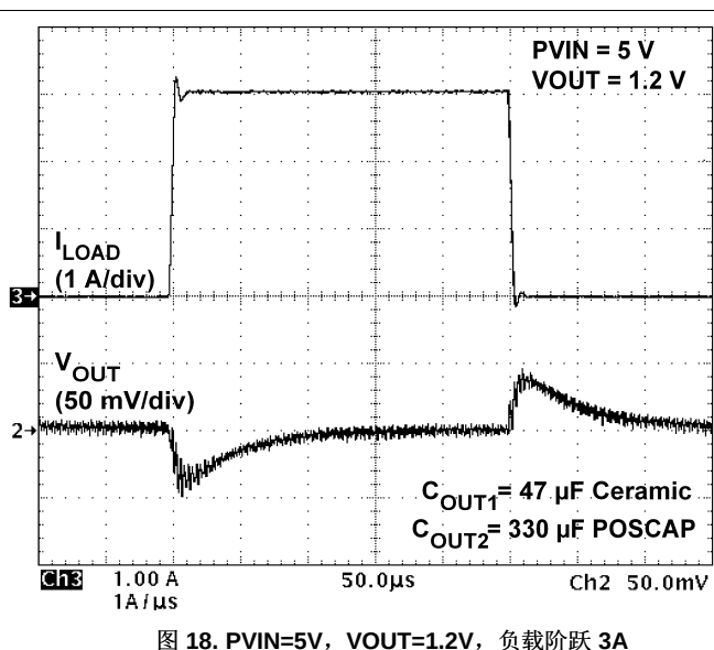
图 18. PV_{IN}=5V , V_{OUT}=1.2V , 负载阶跃 3A
