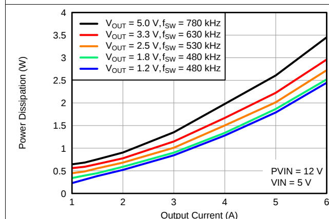
图 13. 功率耗散与输出电流间的关系
