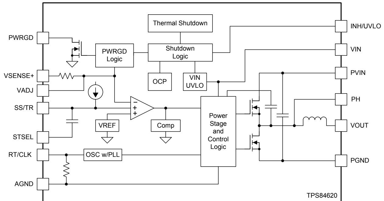
功能方框图
