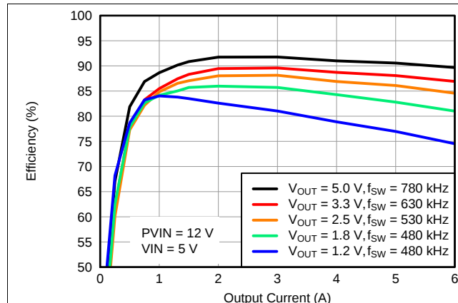
图 11. 效率与输出电流间的关系
