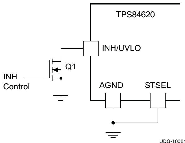
图 30. 典型抑制控制
