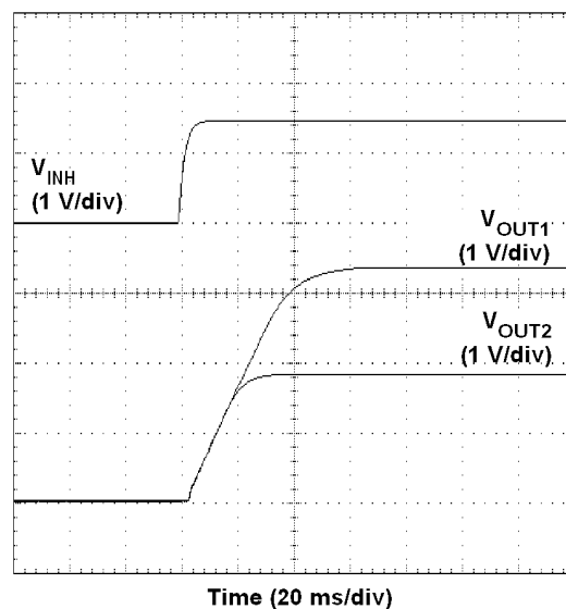
图 40. 同步跟踪波形
