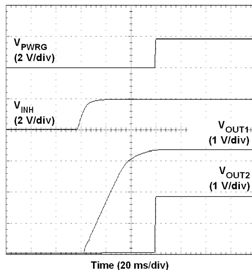
图 38. 排序波形
