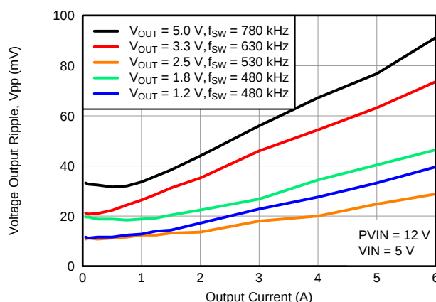
图 12. 电压纹波与输出电流间的关系
