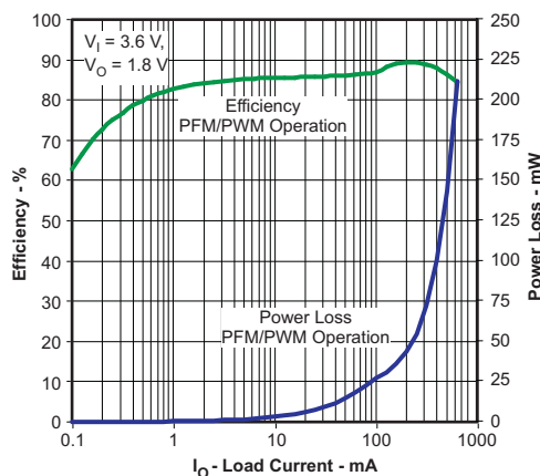
图 2. 效率与 负载电流间的关系
