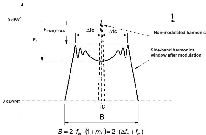
Figure 41. 频率调制正弦波的频谱 随时间正弦变化的波
