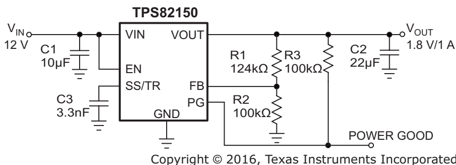
图 5. 1.8-V Output Application
