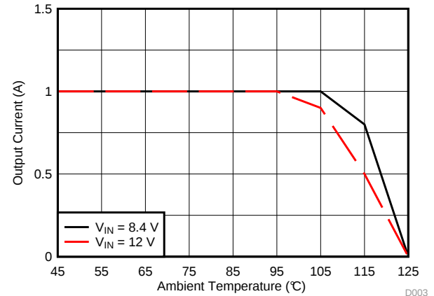
图 19. Thermal Derating, V_{OUT} = 5\text{ V}
