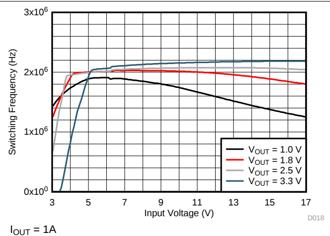
图 23. Switching Frequency
