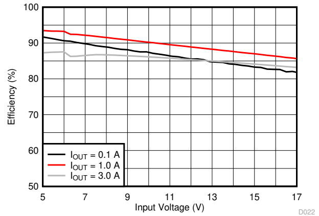
图 8-9. 效率 ( V_{OUT} = 3.3V )
