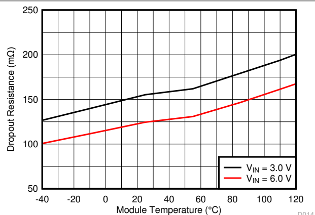
图 6-1. 压降电阻
