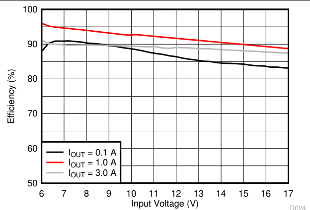
图 8-11. 效率 ( V_{OUT} = 5V )
