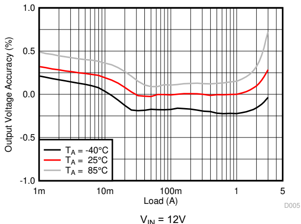
图 8-15. 负载调节
