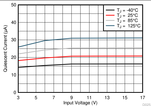
图 6-2. 静态电流
