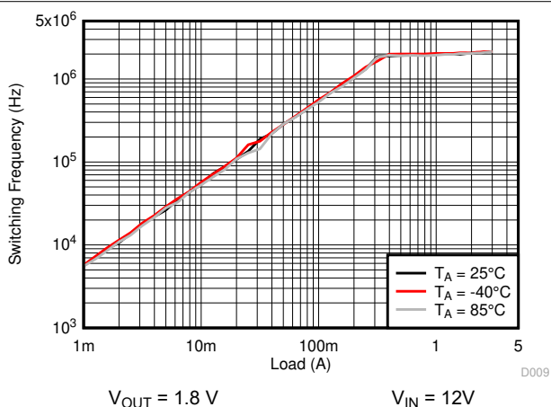
图 8-17. 开关频率
