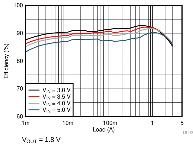
图 8. Efficiency
