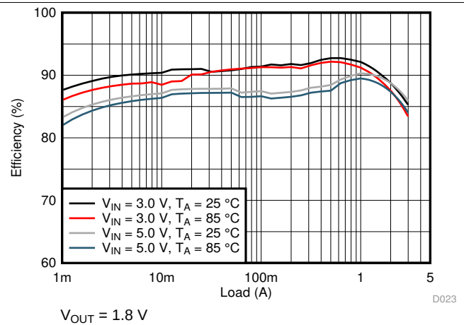
图 9. Efficiency
