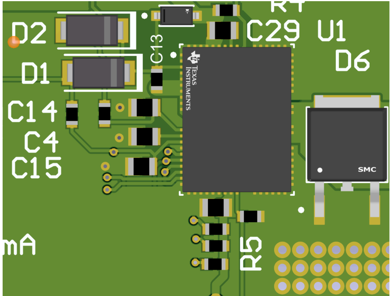
图 9-3. TPS7H6101EVM 的 3D 视图
