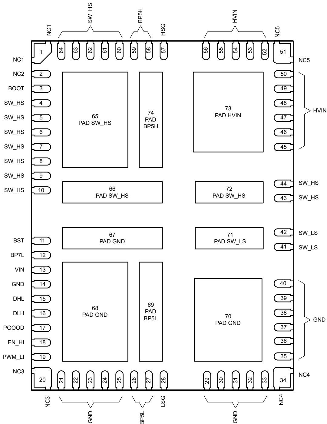
NPR 封装 64 引脚 LGA (顶视图)
