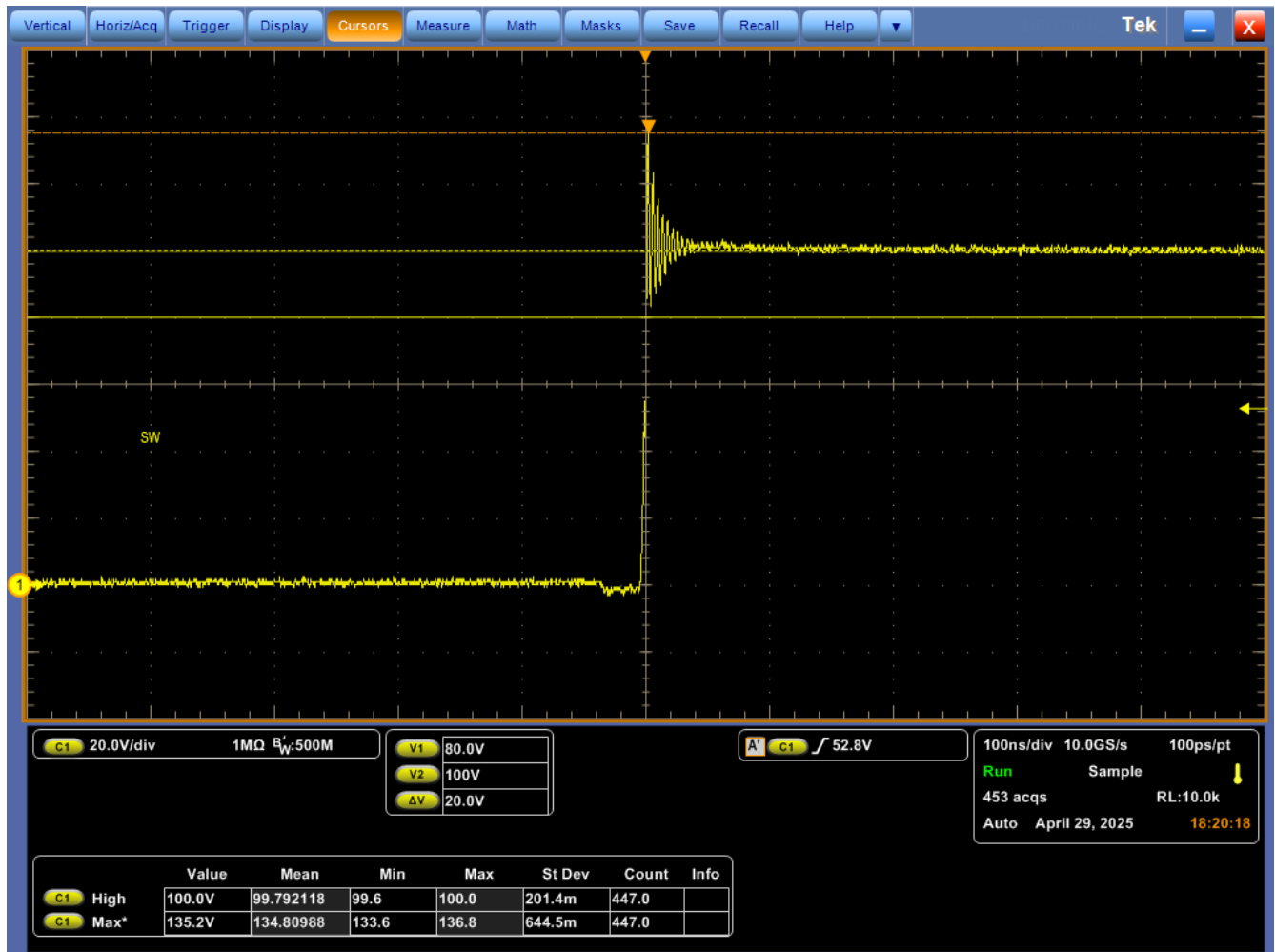
图 9-2. 开关节点上升转换
