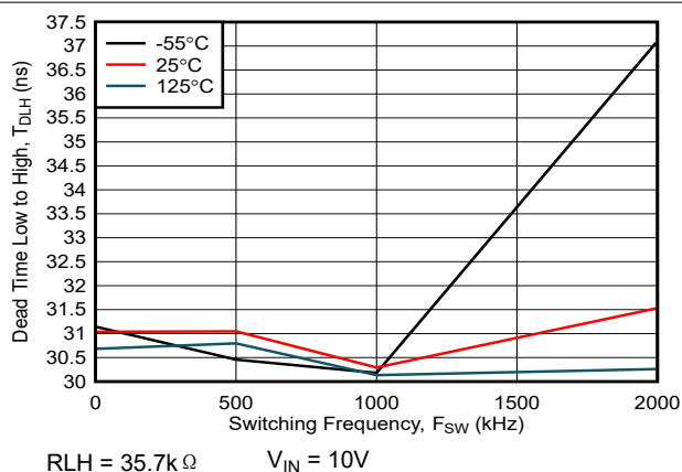
图 6-24. 低电平到高电平死区时间与开关频率间的关系
