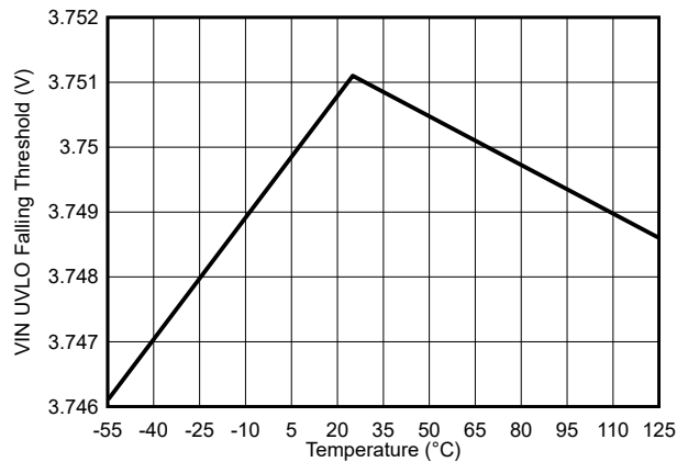
图 7-5. VIN UVLO 下降阈值与温度间的关系
