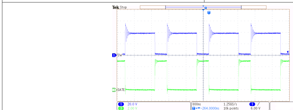
图 9-4. 栅极和开关节点信号
