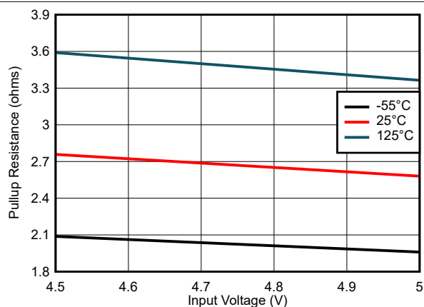
图 7-24. 上拉电阻与输入电压间的关系
