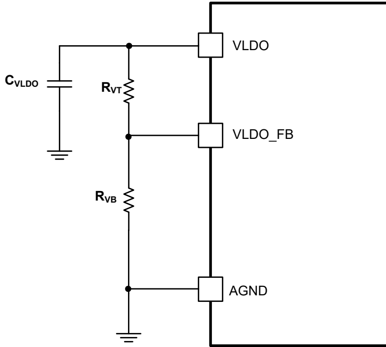
图 8-1. 用于对 VLDO 输出电压进行编程的配置
