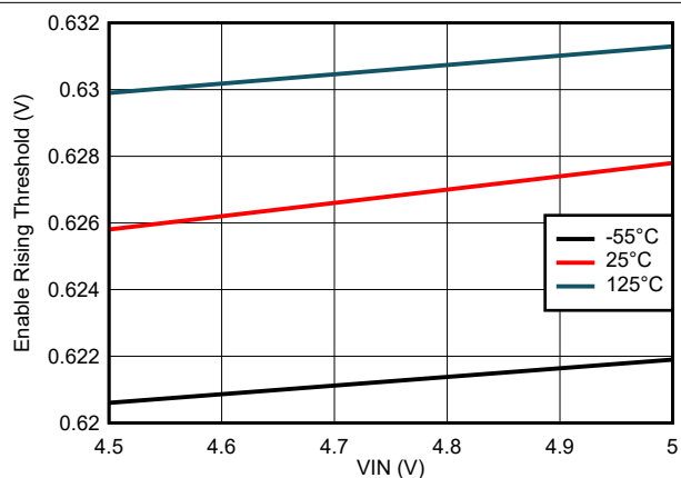
图 7-8. 使能上升阈值与输入电压间的关系
