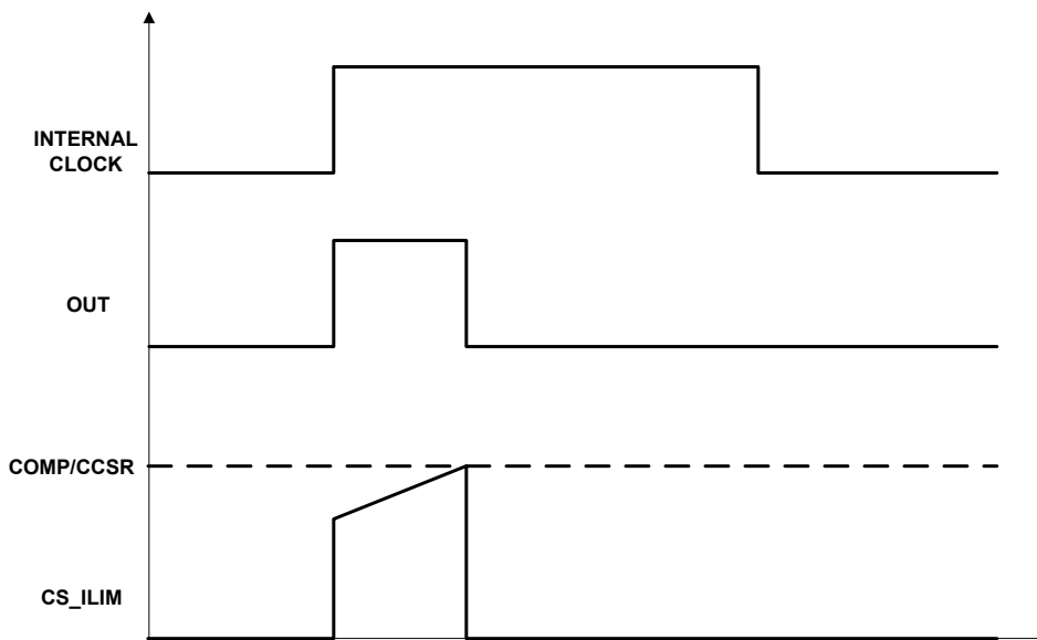
图 8-9. 峰值电流模式控制和 PWM 生成
