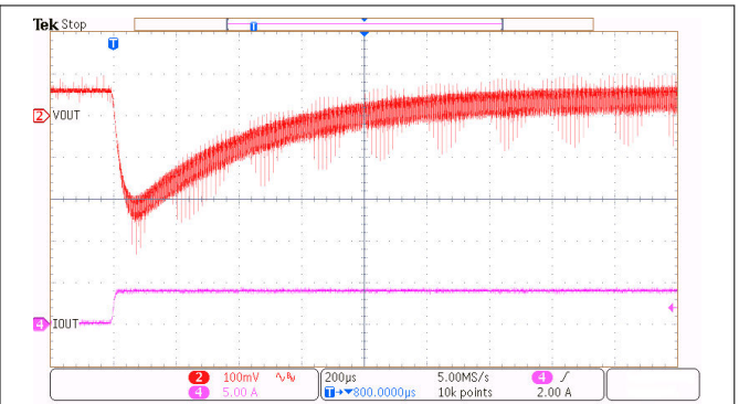
图 9-3. 反激式转换器的 4A 负载阶跃响应
