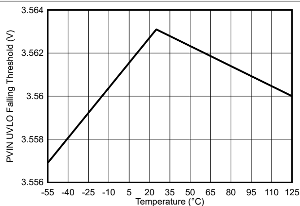
图 7-7. PVIN UVLO 下降阈值与温度间的关系
