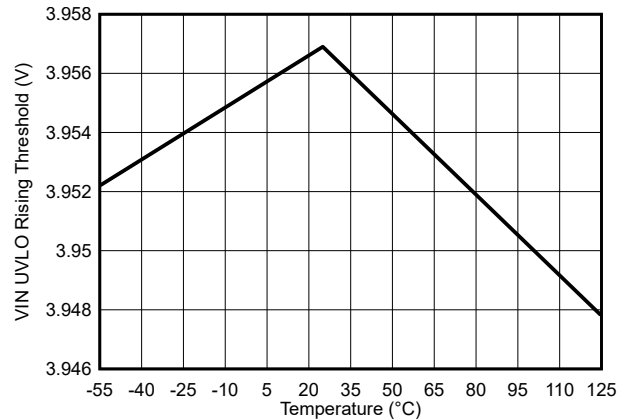
图 7-4. VIN UVLO 上升阈值与温度间的关系
