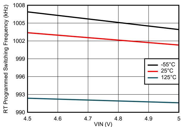
图 7-16. 开关频率与输入电压间的关系
