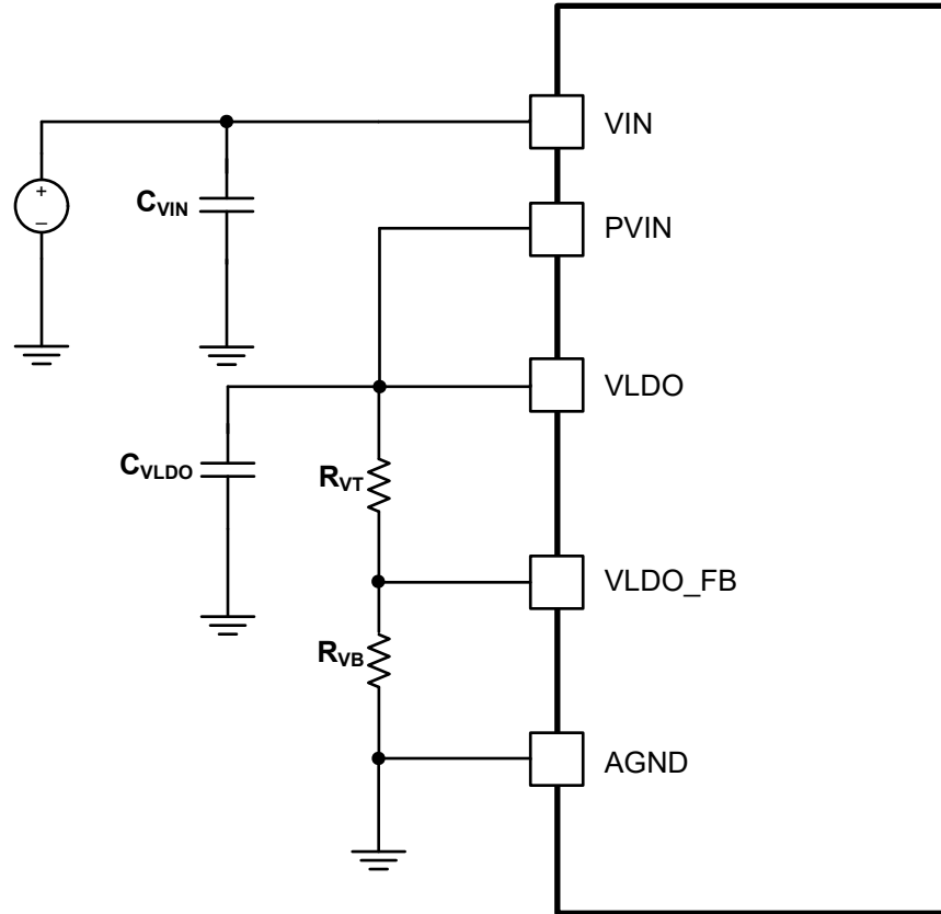
图 8-3. PVIN 至 VLDO 连接的配置
