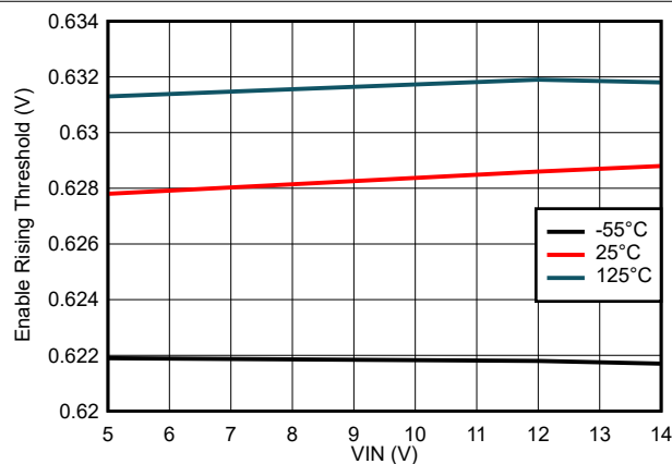
图 7-9. 使能上升阈值与输入电压间的关系
