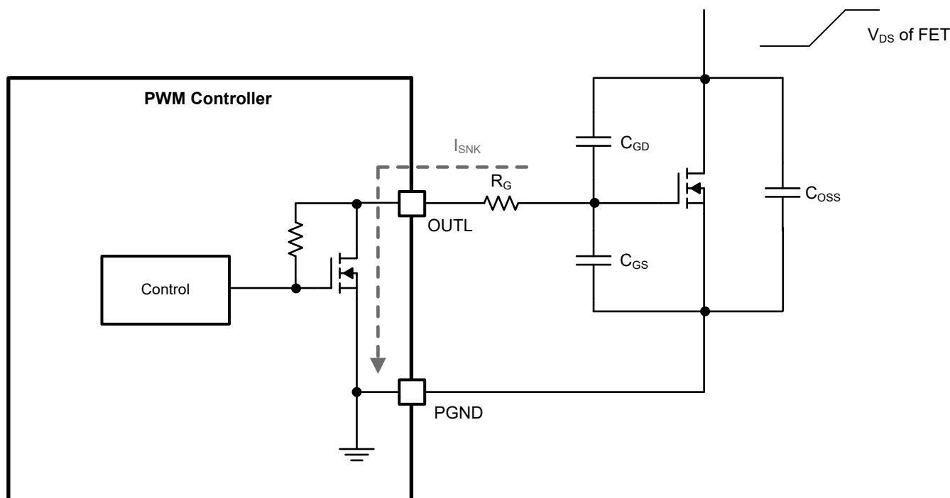
图 8-10. 未上电的电压钳位
