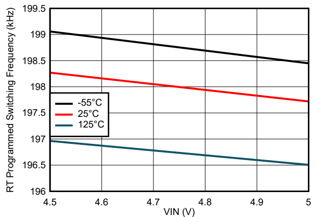
图 7-12. 开关频率与输入电压间的关系
