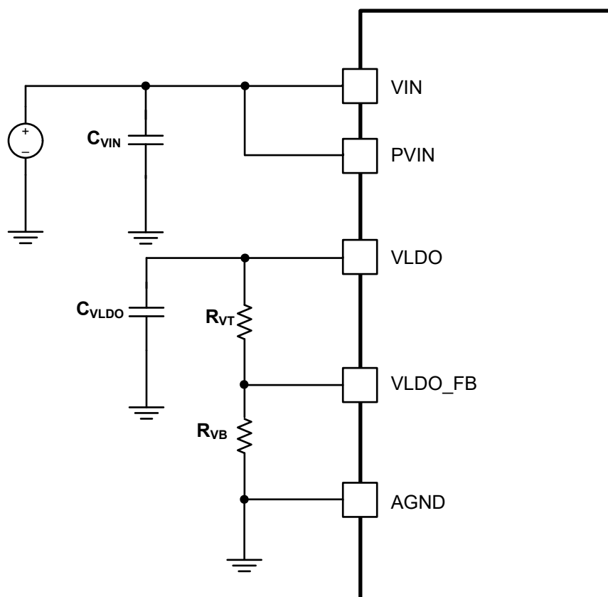
图 8-2. PVIN 到 VIN 连接的配置
