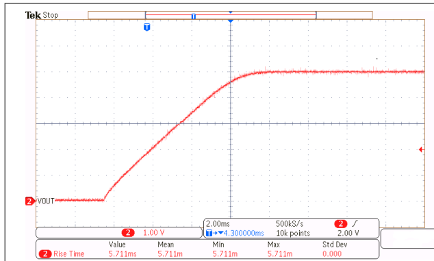
图 9-2. 反激式转换器的 V_{OUT} 启动
