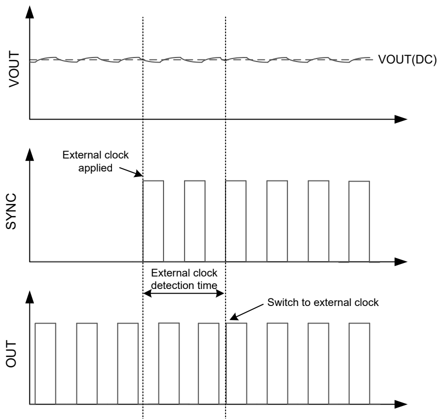
图 8-7. 内部至外部时钟转换
