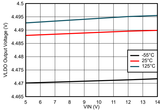
图 7-1. 内部线性稳压器输出电压与输入电压间的关系
