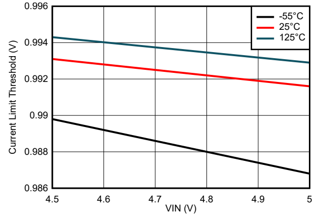
图 7-22. 电流限制阈值与输入电压间的关系
