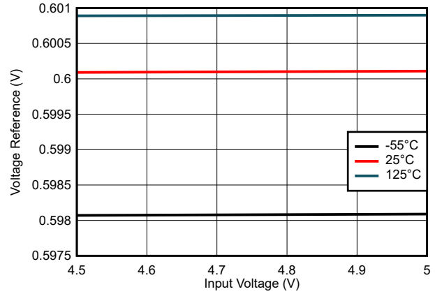
图 7-20. 内部电压基准与输入电压间的关系
