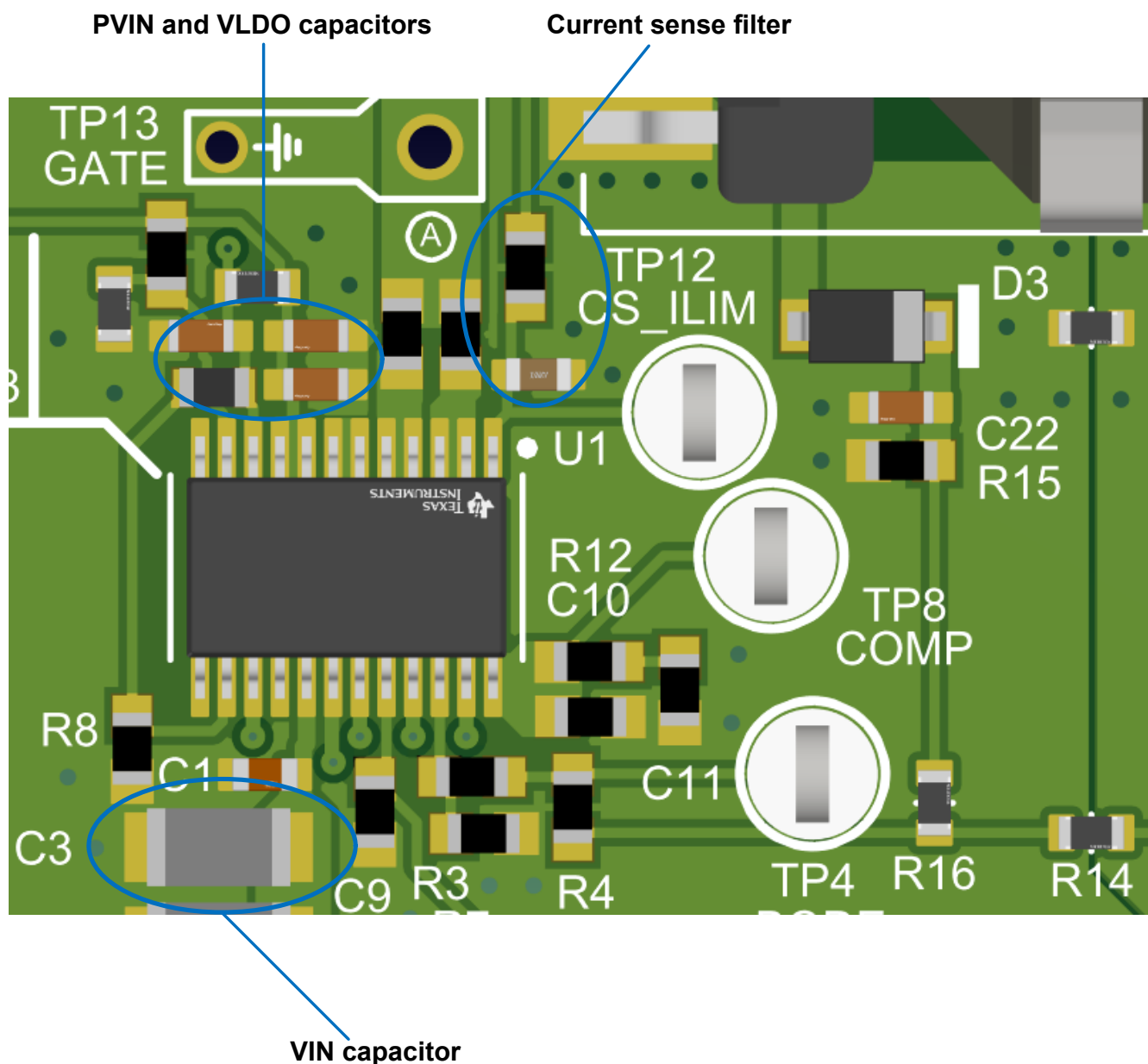
图 9-5. TPS7H5020FLYEVM 的 3D 布局视图
