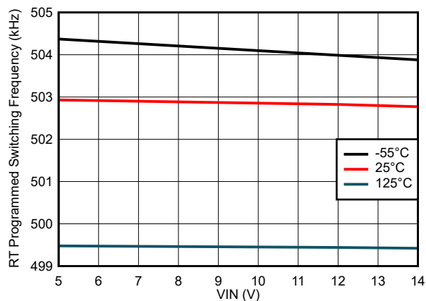
图 7-15. 开关频率与输入电压间的关系
