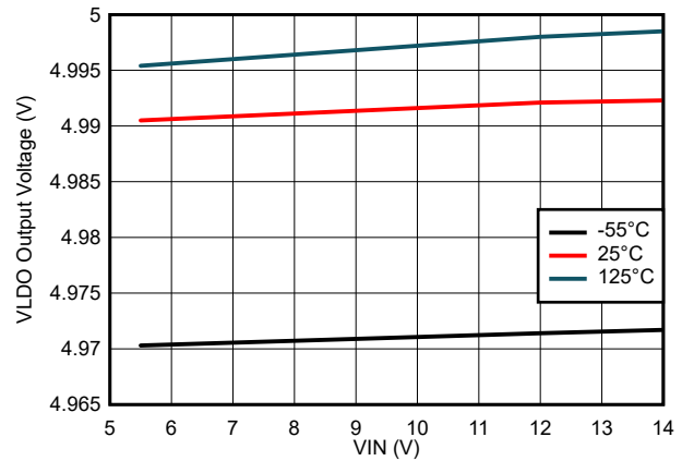
图 7-2. 内部线性稳压器输出电压与输入电压间的关系
