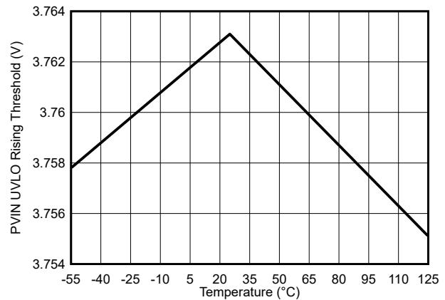
图 7-6. PVIN UVLO 上升阈值与温度间的关系
