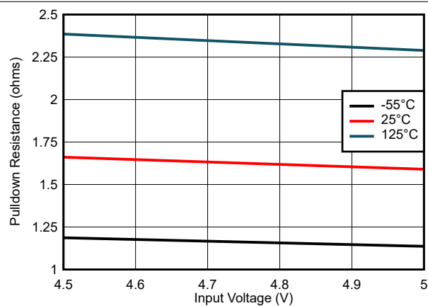
图 7-27. 下拉电阻与输入电压间的关系
