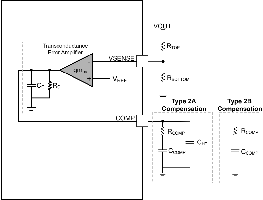
图 8-11. TPS7H502x 频率补偿选项
