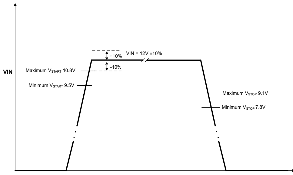
图 8-5. VIN = 12V 时双电阻配置的启动值和 UVLO 值
