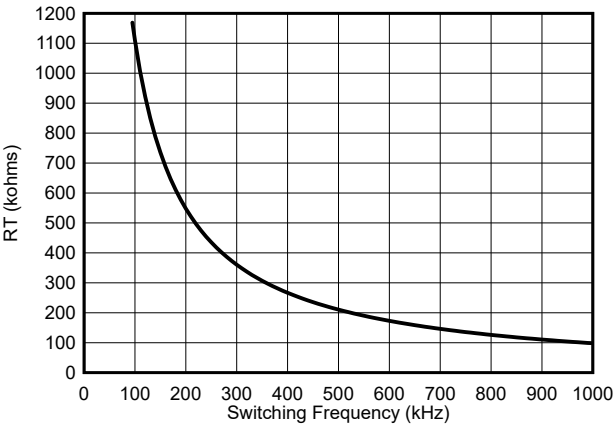
图 8-6. RT 与开关频率间的关系
