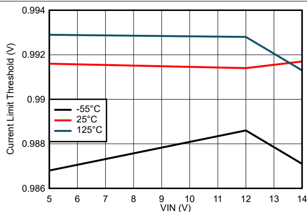
图 7-23. 电流限制阈值与输入电压间的关系
