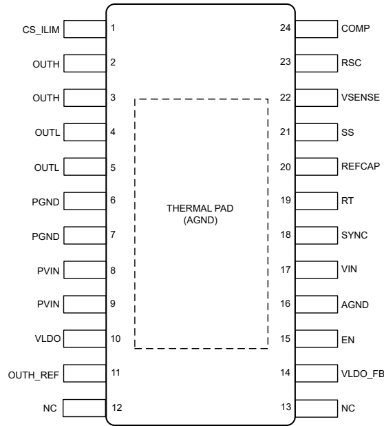
图 6-1. PWP 封装 散热焊盘的 24 引脚带 HTSSOP (顶视图)
