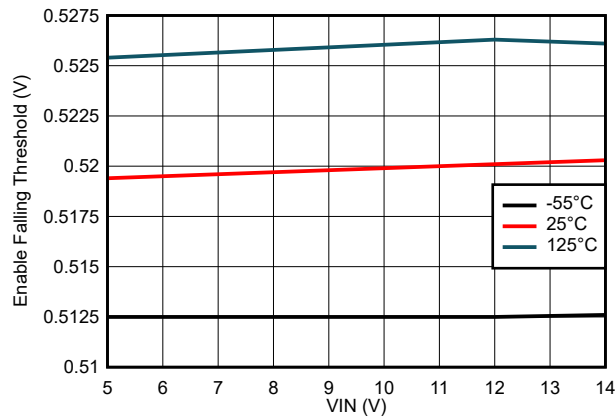
图 7-11. 使能下降阈值与输入电压间的关系
