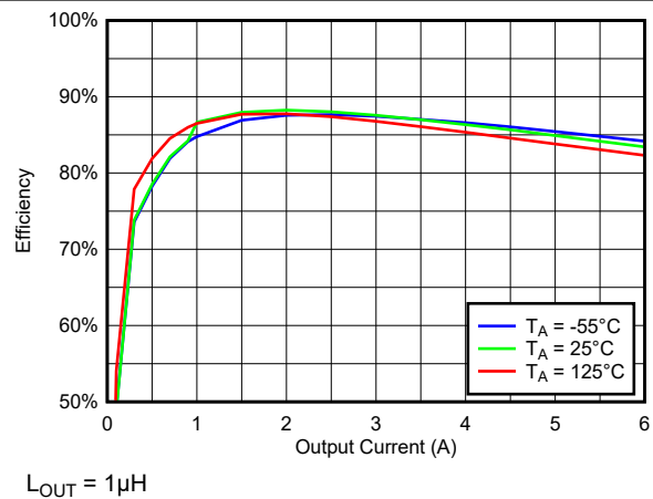
图 7-20. 1MHz、 V_{IN} = 5V 、 V_{OUT} = 1.8V 时整个温度范围内的效率与负载间的关系
