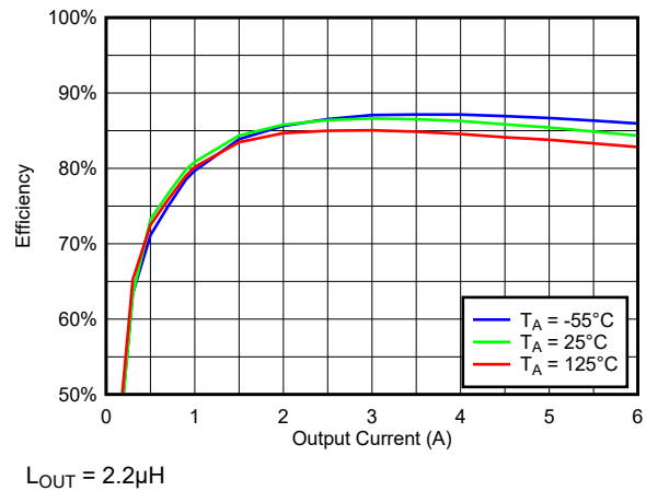
图 7-18. 500kHz、 V_{IN} = 12V 、 V_{OUT} = 1.8V 时整个温度范围内的效率与负载间的关系
