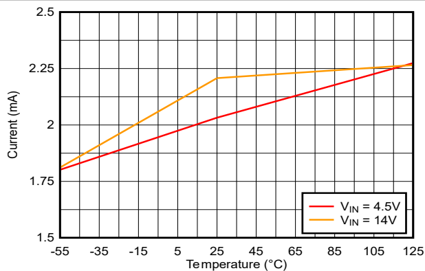
图 7-26. V_{IN} 关断电流与温度间的关系
