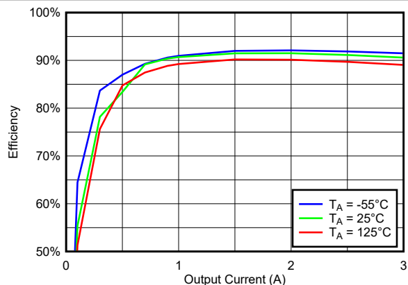
图 7-25. TPS7H4013 在 500kHz、 V_{IN} = 5V 、 V_{OUT} = 1.8V 时整个温度范围内的效率与负载间的关系
