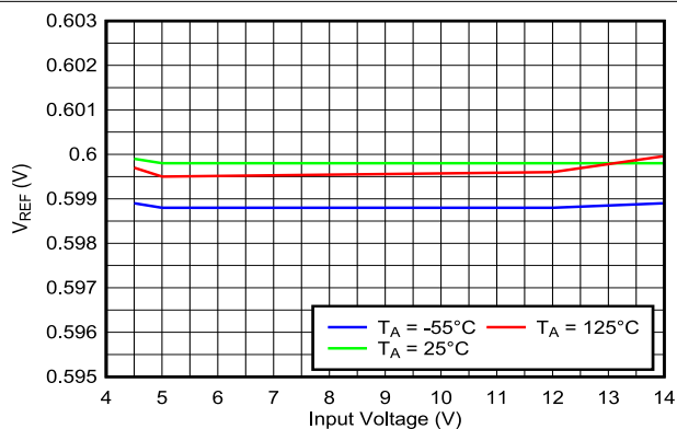
图 7-30. V_{REF} 与输入电压间的关系
