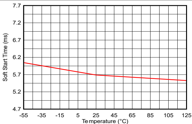
图 6-56. 软启动时间与温度间的关系
