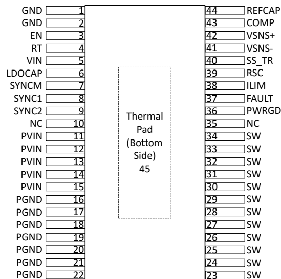
图 5-2. DDW 封装，44 引脚 HTSSOP (顶视图)
