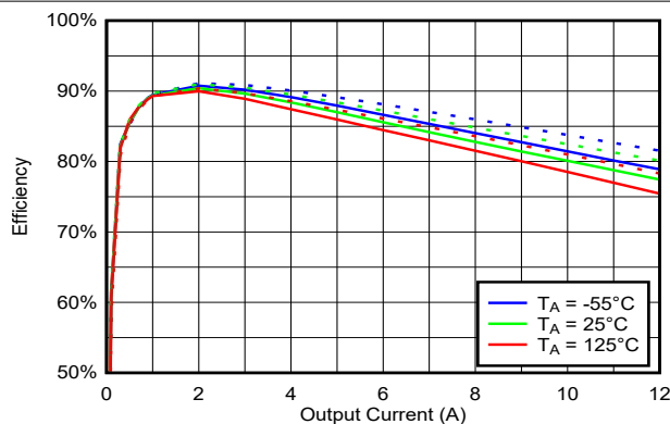
图 6-17. 500kHz、 V_{IN} = 12V 、 V_{OUT} = 3.3V 时整个温度范围内的效率与负载间的关系
