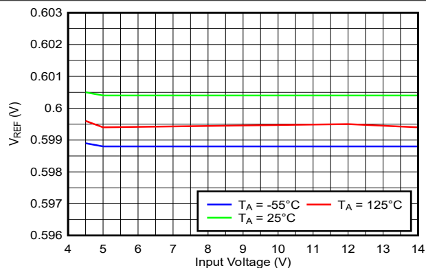
图 6-31. V_{REF} 与输入电压间的关系
