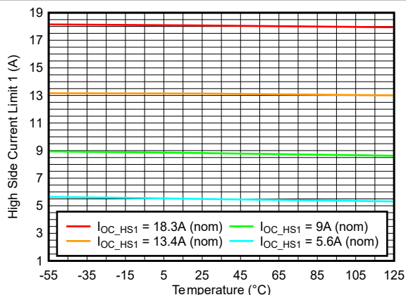
图 6-40. 高侧电流限值阈值 1 ( I_{OC\_HS1} ) 与温度间的关系
