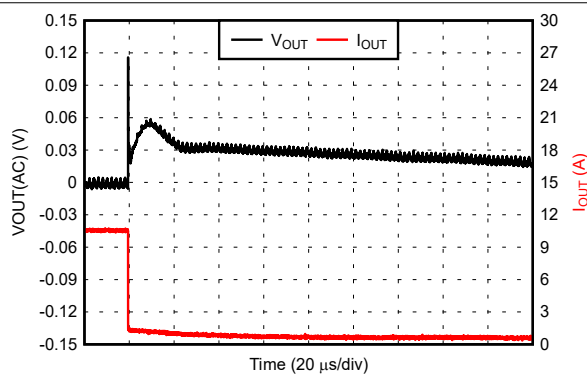
图 6-64. 负载阶跃: 10.6A 至 0.6A
