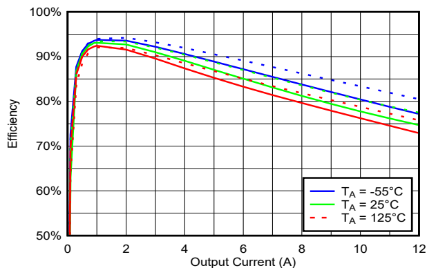
图 6-6. V_{IN} = 12V 、 1MHz 时 V_{OUT} 范围内的效率与负载间的关系
