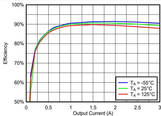
图 6-23. 500kHz、 V_{IN} = 12V 、 V_{OUT} = 5V 时 整个温度范围内的低电流效率与负载间的关系
