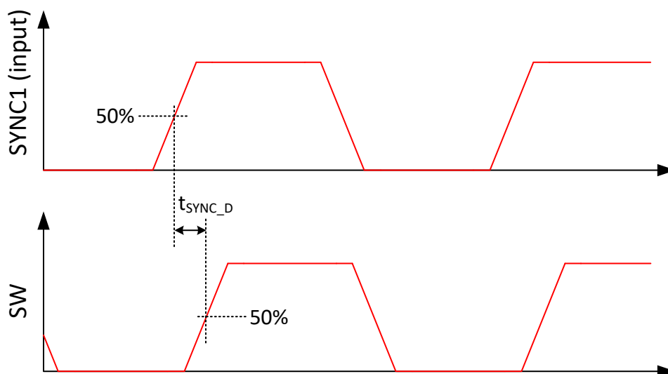
图 7-5. SYNC1 到 SW 延迟：非反相同步
