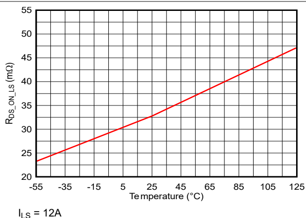
图 6-62. 低侧 FET 电阻与温度间的关系
