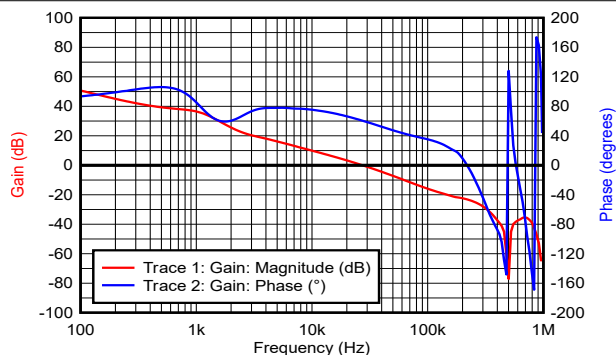
图 9-4. 波特图
