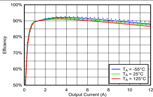
图 6-19. 1MHz、 V_{IN} = 5V 、 V_{OUT} = 2.5V 时整个温度范围内的效率与负载间的关系
