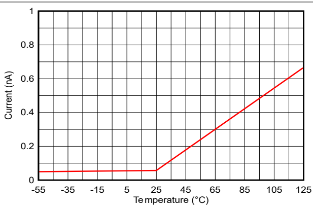
图 6-28. VIN 静态电流 (非开关) 与温度间的关系
