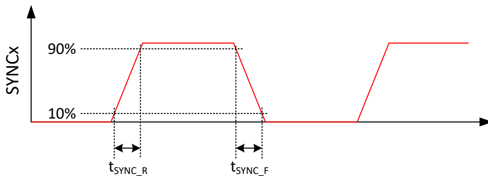
图 7-3. SYNCx 上升和下降时间
