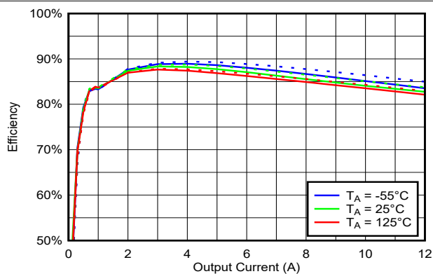
图 6-20. 1MHz、 V_{IN} = 5V 、 V_{OUT} = 1.8V 时整个温度范围内的效率与负载间的关系
