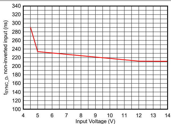
图 6-48. SYNC1 至 SW 延迟 (同相输入) 与输入电压间的关系
