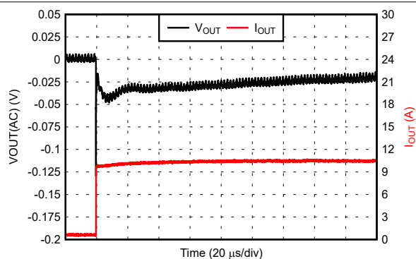
图 6-63. 负载阶跃: 0.6A 至 10.5A
