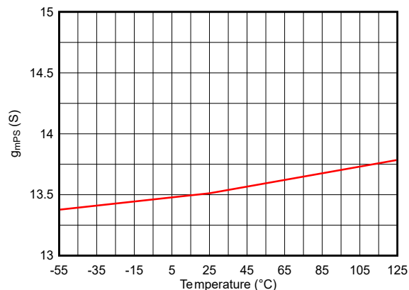
图 6-37. I_{OC\_HS1} = 13.4A 时的功率级跨导 ( g_{mps} ) 与温度间的关系
