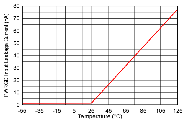
图 6-57. 电源正常状态泄漏与温度间的关系
