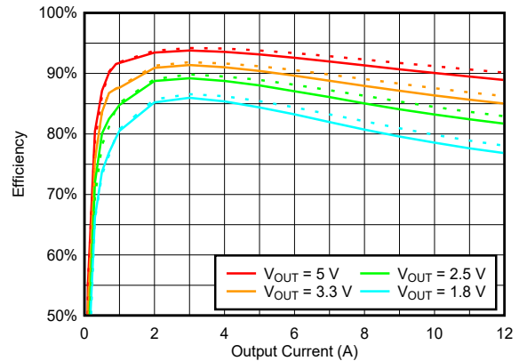
图 6-4. V_{IN} = 12V 、500kHz 时 V_{OUT} 范围内的效率与负载间的关系
