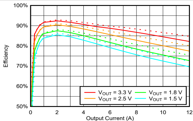
图 6-5. V_{IN} = 5V 、 1MHz 时 V_{OUT} 范围内的效率与负载间的关系
