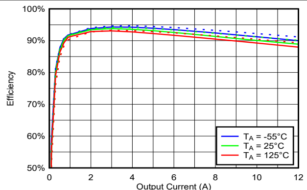
图 6-14. 500kHz、 V_{IN} = 5V 、 V_{OUT} = 1.8V 时整个温度范围内的效率与负载间的关系
