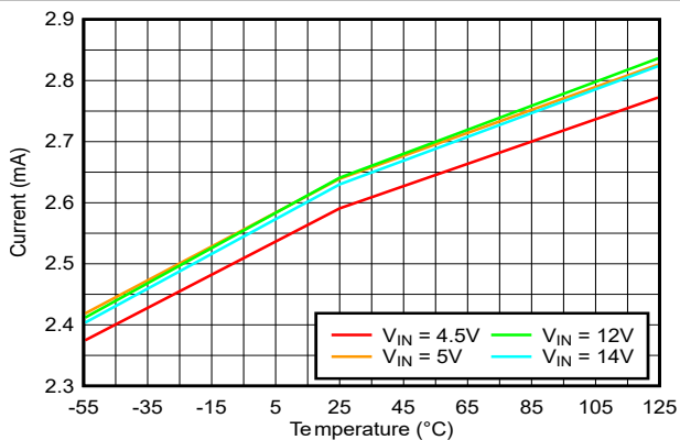
图 6-28. VIN 静态电流 (非开关) 与温度间的关系
