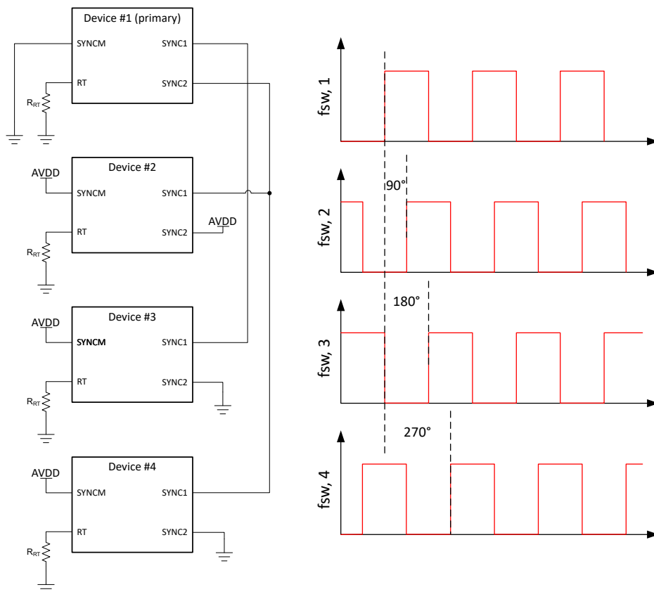
图 8-11. 4 个器件并行工作
