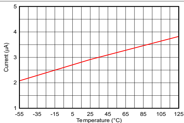
图 6-27. PVIN 关断电流与温度间的关系
