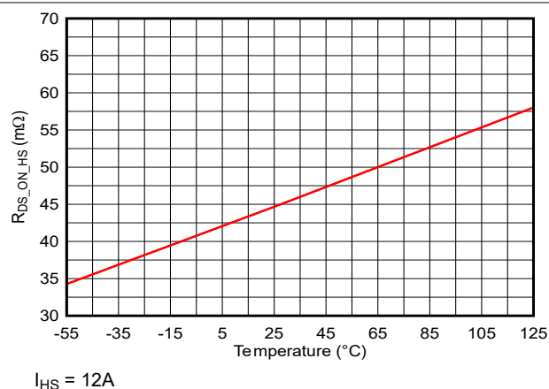
图 6-61. 高侧 FET 电阻与温度间的关系
