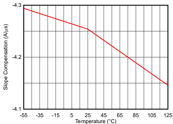
图 6-44. 500kHz 下斜率补偿与温度间的关系
