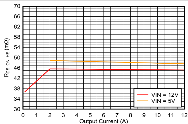
图 6-59. 高侧 FET 电阻与电流间的关系
