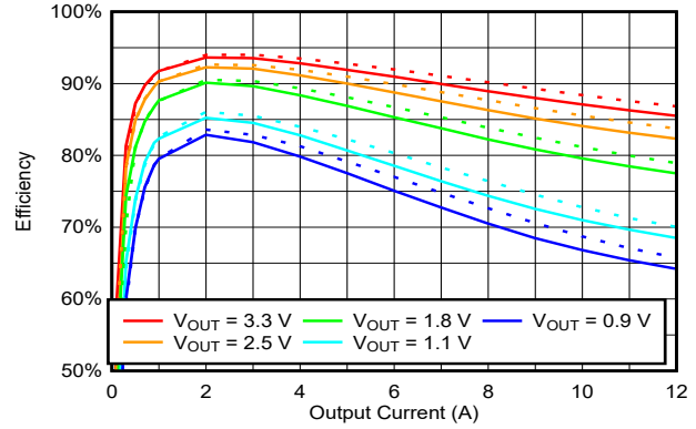
图 6-2. V_{IN} = 12V 、100kHz 时 V_{OUT} 范围内的效率与负载间的关系
