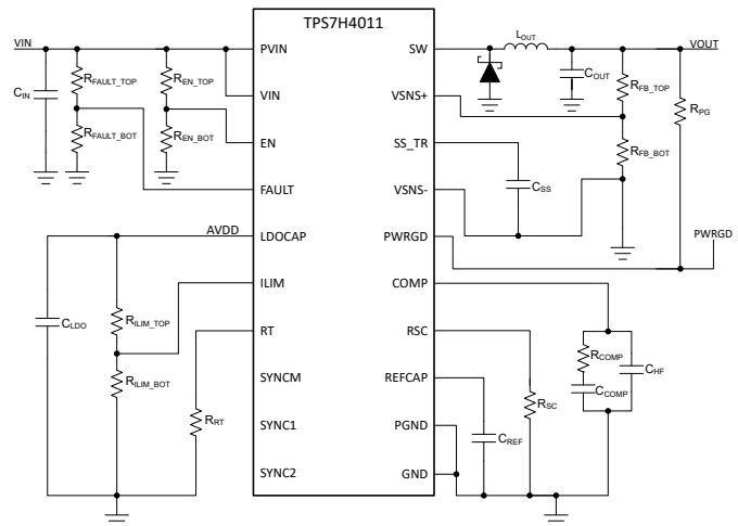
简化版原理图
