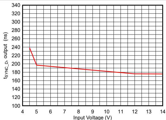
图 6-52. SYNC1 至 SW 延迟 (输出) 与输入电压间的关系
