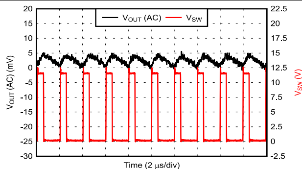
图 9-3. 开关节点波形和输出电压纹波
