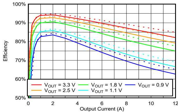
图 6-1. V_{IN} = 5V 、100kHz 时 V_{OUT} 范围内的效率与负载间的关系
