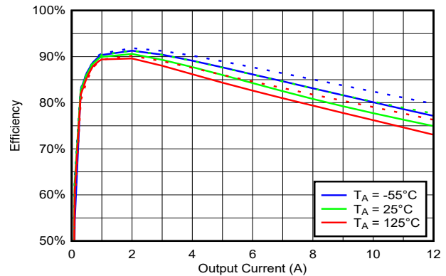
图 6-12. 100kHz、 V_{IN} = 12V 、 V_{OUT} = 1.8V 时整个温度范围内的效率与负载间的关系
