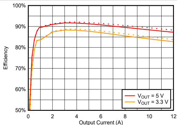
图 6-6. V_{IN} = 12V 、 1MHz 时 V_{OUT} 范围内的效率与负载间的关系
