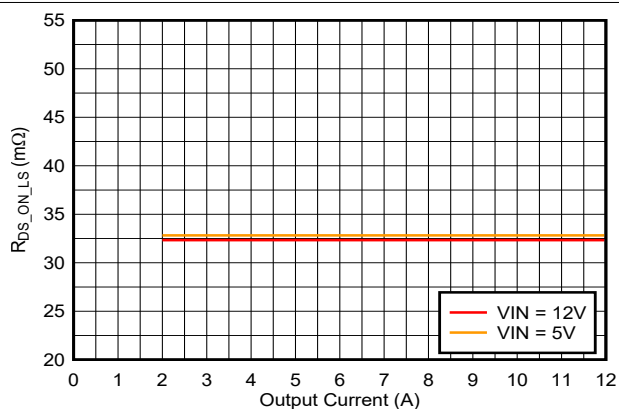
图 6-60. 低侧 FET 电阻与电流间的关系
