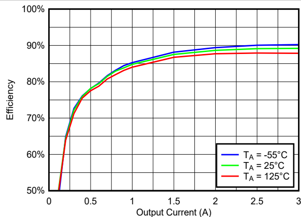
图 6-24. 500kHz、 V_{IN} = 12V 、 V_{OUT} = 2.5V 时 整个温度范围内的低电流效率与负载间的关系
