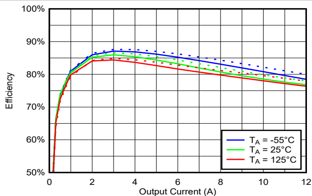
图 6-18. 500kHz、 V_{IN} = 12V 、 V_{OUT} = 1.8V 时整个温度范围内的效率与负载间的关系
