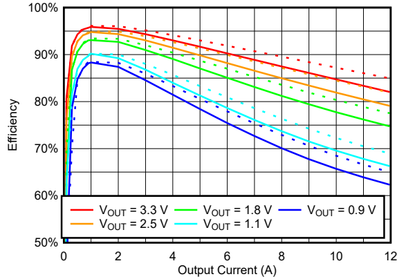
图 6-1. V_{IN} = 5V 、100kHz 时 V_{OUT} 范围内的效率与负载间的关系
