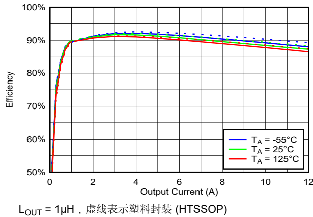
图 6-21. 1MHz、 V_{IN} = 12V 、 V_{OUT} = 5V 时整个温度范围内的效率与负载间的关系
