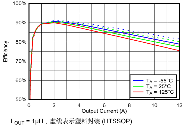
图 6-19. 1MHz、 V_{IN} = 5V 、 V_{OUT} = 2.5V 时整个温度范围内的效率与负载间的关系
