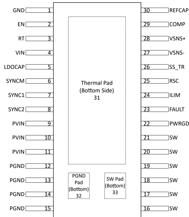
图 5-1. HLB 封装，30 引脚 CFP (顶视图)
