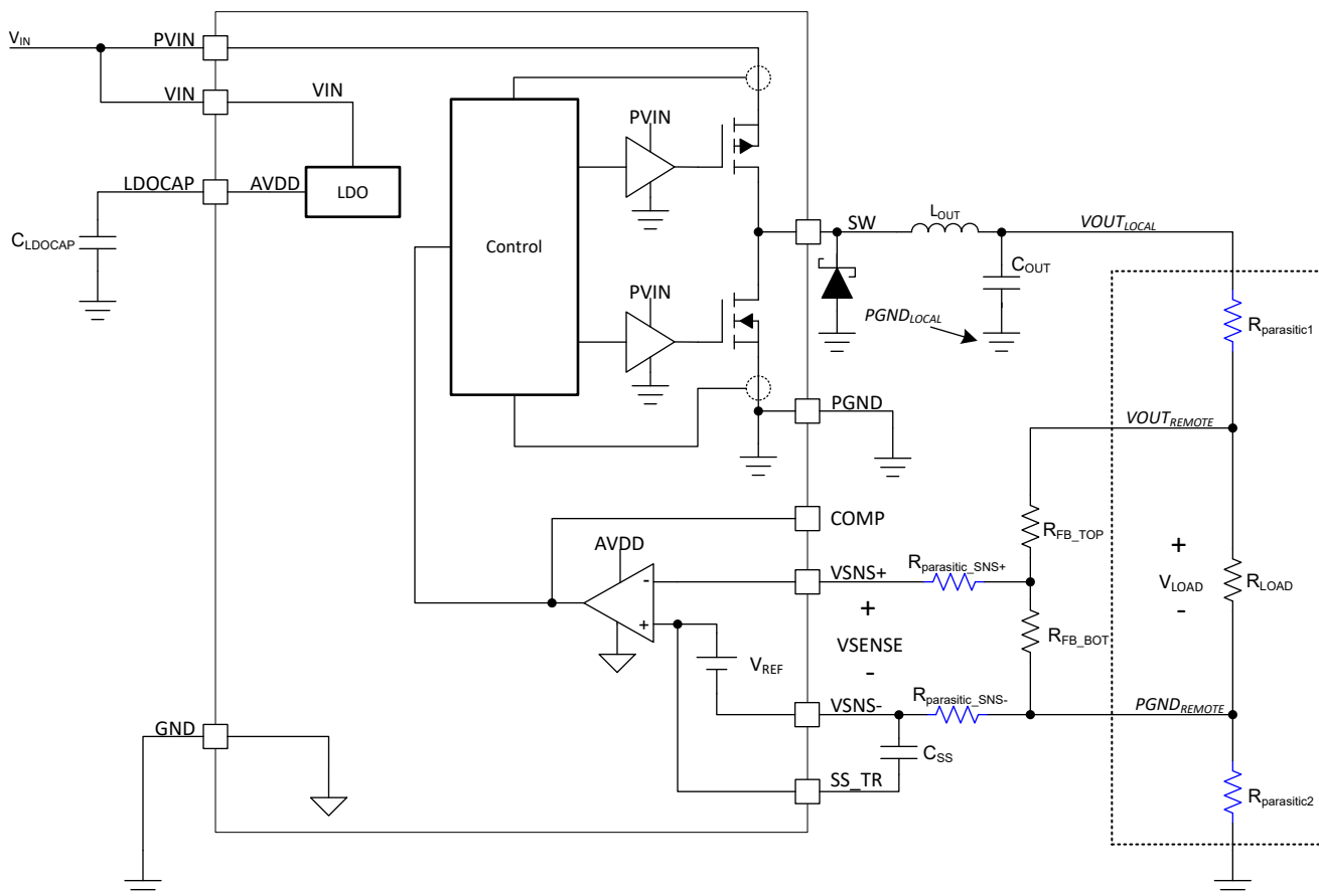
图 8-2. 遥感方框图
