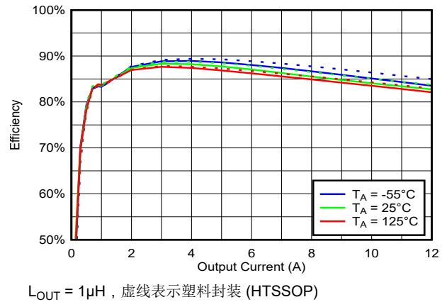
图 6-22. 1MHz、 V_{IN} = 12V 、 V_{OUT} = 3.3V 时整个温度范围内的效率与负载间的关系
