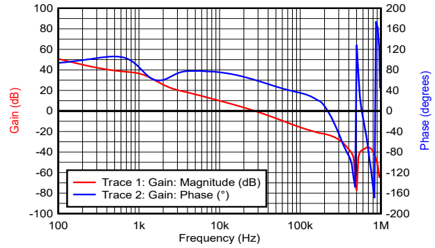
图 9-4. 波特图
