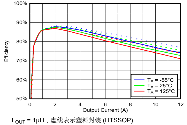
图 6-20. 1MHz、 V_{IN} = 5V 、 V_{OUT} = 1.8V 时整个温度范围内的效率与负载间的关系
