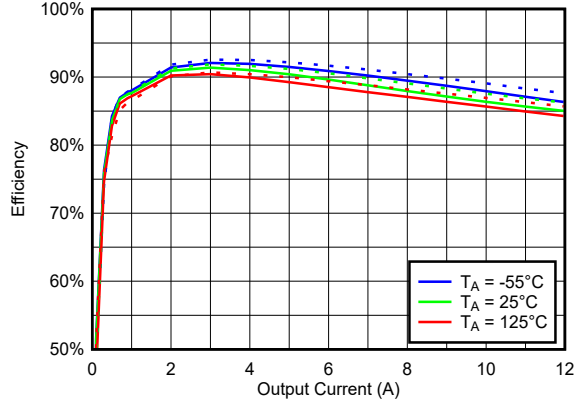
图 6-17. 500kHz、 V_{IN} = 12V 、 V_{OUT} = 3.3V 时整个温度范围内的效率与负载间的关系
