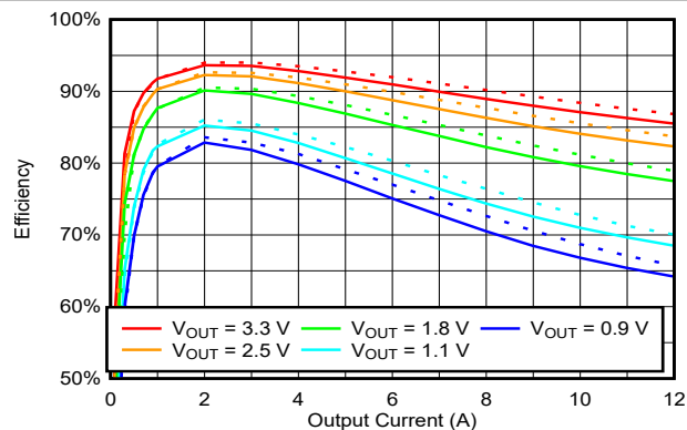
图 6-2. V_{IN} = 12V 、 100kHz 时 V_{OUT} 范围内的效率与负载间的关系
