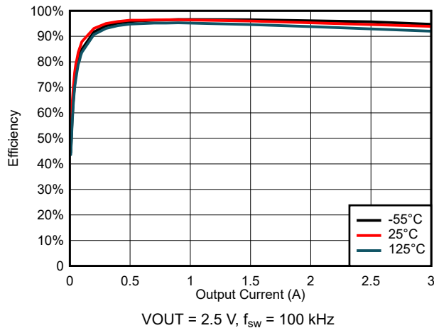
图 6-49. Efficiency fo VIN = 5.5 V
