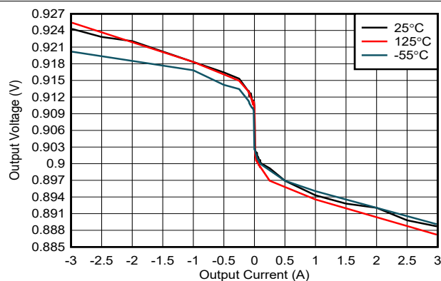
图 6-2. Output Voltage vs Output Current
