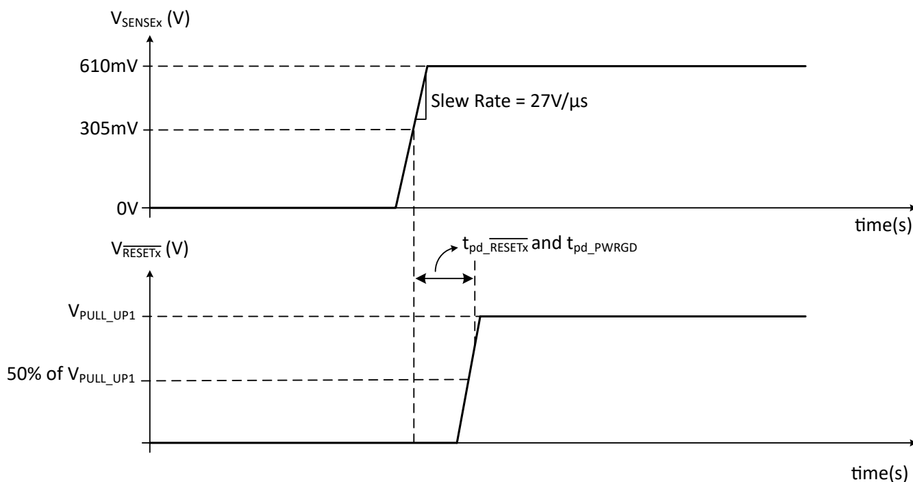
图 7-2. \overline{RESETx} 和 \overline{PWRGD} 传播延迟 ( t_{pd\_RESETx} 和 t_{pd\_PWRGD} ) 时间测量
