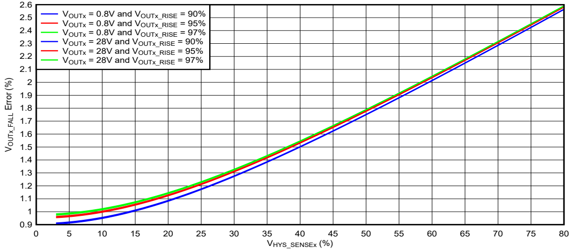
图 8-8. V_{OUTx\_FALL} 绝对误差与 V_{HYS\_SENSEx} 间的关系
