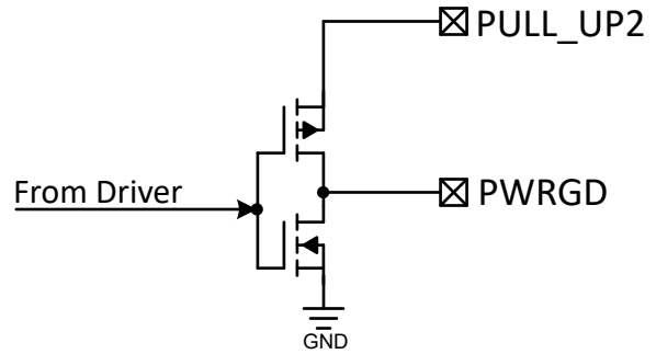
图 8-11. UV 通道类型的 PWRGD 推挽输出级
