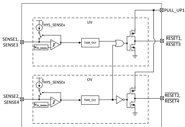
图 8-9. 当 MODE=1 时 TPS7H3024 的窗口比较器
