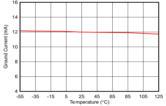
图 6-8. 接地电流与温度间的关系
