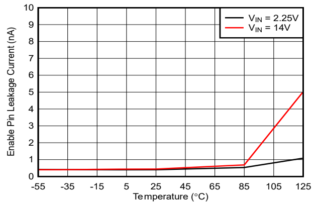
图 6-12. 使能引脚漏电流与温度间的关系
