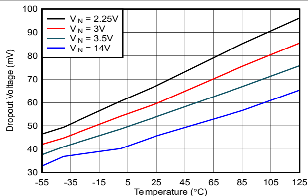
图 6-4. 压降电压与温度间的关系
