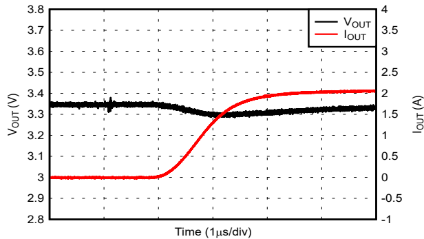
图 6-23. 负载阶跃: 0A 至 2A 且 V_{IN} = 5V
