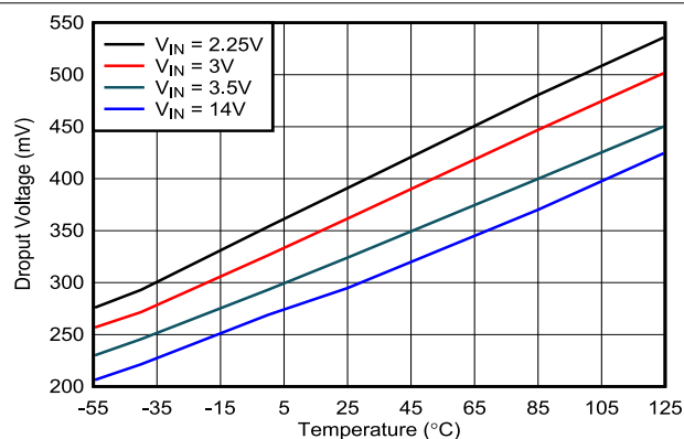
图 6-3. 压降电压与温度间的关系
