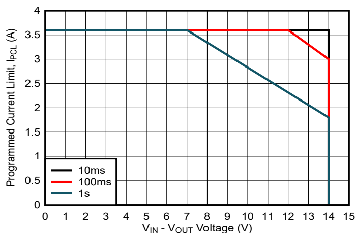
图 9-2. 可编程电流限制保护区域
