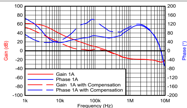
图 6-15. 增益和相位裕度与频率间的关系 (波特图)
