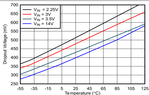
图 6-2. 压降电压与温度间的关系
