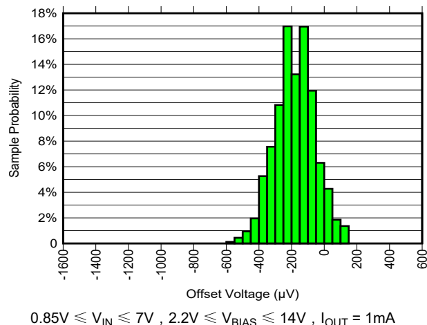
图 6-48. T_A = 25^{\circ}C 时的输出失调电压分布
