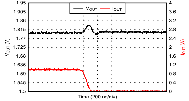
压摆率 = 8.1A/\mu s I_{OUT} 仅仅是步进变化的电流, 未显示并联的 0.5A 负载
