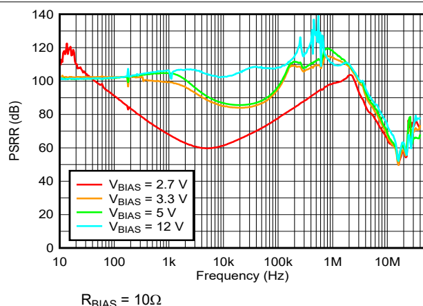
图 6-13. 使用 RC 时在不同偏置电压下 PSRR_{BIAS} 与频率间的关系
