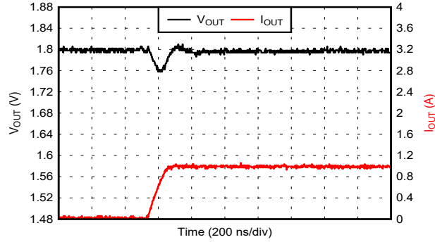
压摆率 = 8.5A/\mu s I_{OUT} 仅仅是步进变化的电流, 未显示并联的 0.5A 负载
