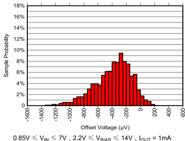
图 6-49. T_A = 125^{\circ}C 时的输出失调电压分布
