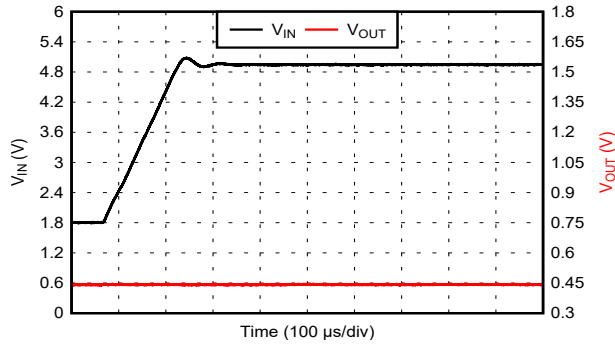
压摆率: 20.2V/ms V_{OUT} = 0.4V 图 6-62. 线路阶跃: 1.8V 至 5V , 其中 I_{OUT} = 1.5A
