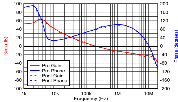
图 9-12. 波特图：器件 2， I_{OUT} = 100\text{mA}
