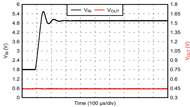
压摆率 = 84.0V/ms V_{OUT} = 0.4V 图 6-64. 线路阶跃: 1.8V 至 5V , 其中 I_{OUT} = 1mA
