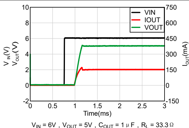
图 5-22. 加电波形
