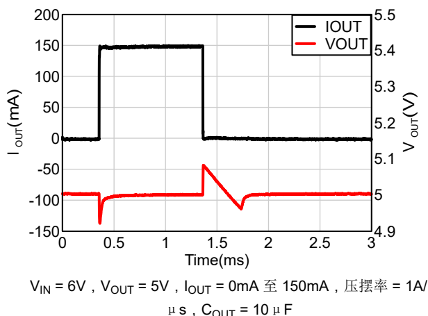
图 5-20. 负载瞬态响应与时间之间的关系
