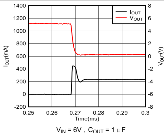
图 5-21. 短路电流与时间之间的关系
