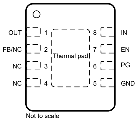
图 4-2. DRB 封装，8 引脚 VSON（顶视图）
