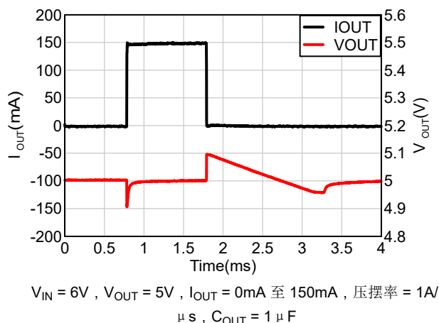
图 5-19. 负载瞬态响应与时间之间的关系
