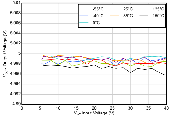
图 5-1. 输出电压与温度间的关系
