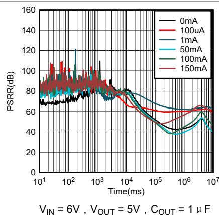
图 5-24. 波纹抑制与频率
