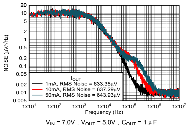
图 5-42. 噪声与负载电流间的关系
