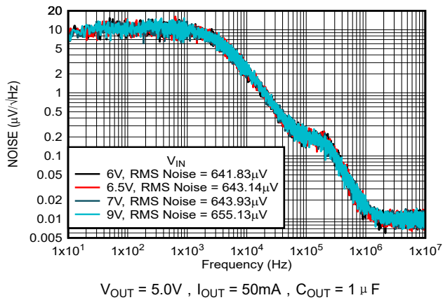
图 5-43. 噪声与输入电源间的关系
