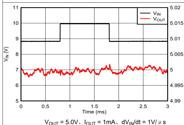
图 7-8. V_{IN} 线路瞬态 (8.8V 至 10V)
