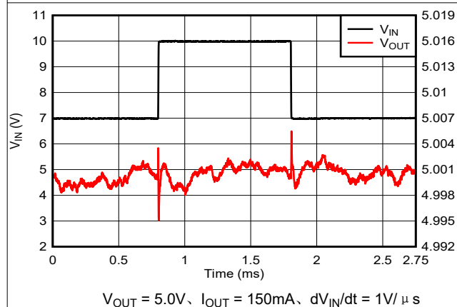
图 5-23. V_{IN} 线路瞬态 (7V 至 10V)
