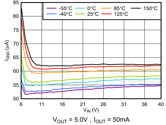
图 5-14. I_{GND} 与 V_{IN} 间的关系
