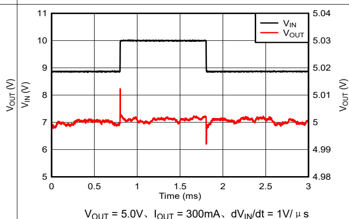
图 7-9. V_{IN} 线路瞬态 (8.8V 至 10V)
