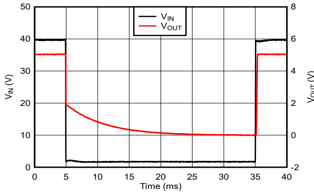
图 7-16. 欠压瞬态 (40V 至 1.7V)
