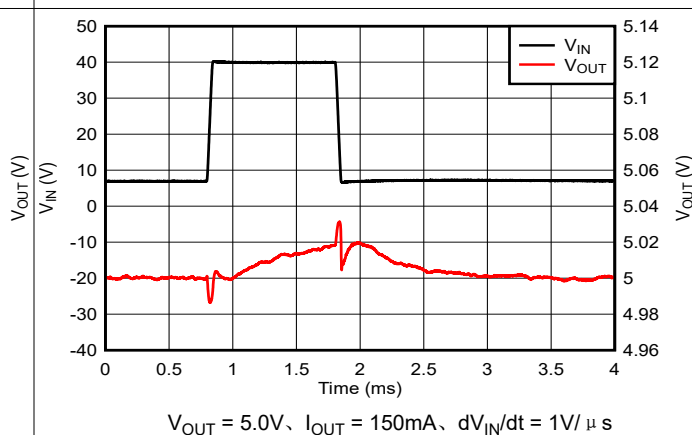
图 7-7. V_{IN} 线路瞬态 (7V 至 40V)
