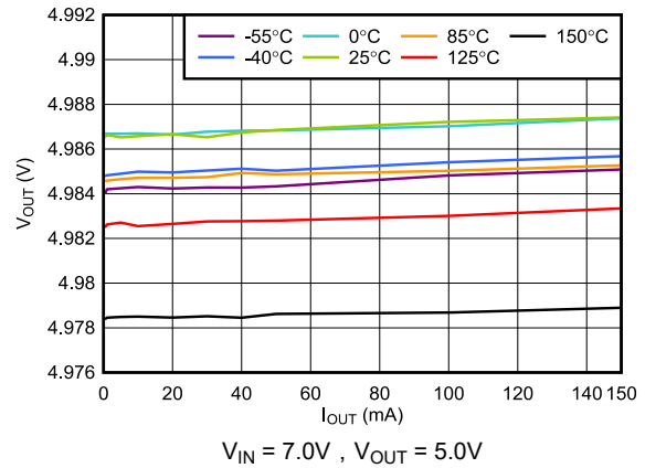
图 5-6. V_{OUT} 与 I_{OUT} 间的关系
