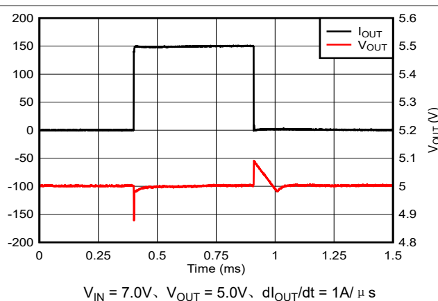
图 7-13. 负载瞬态 (1mA 至 150mA)
