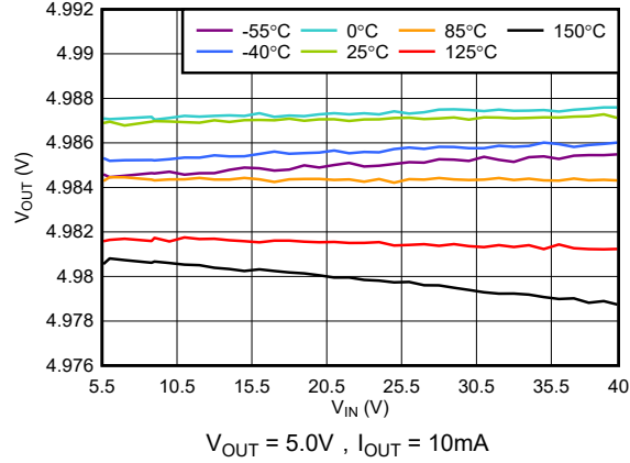
图 5-1. V_{OUT} 与 V_{IN} 间的关系
