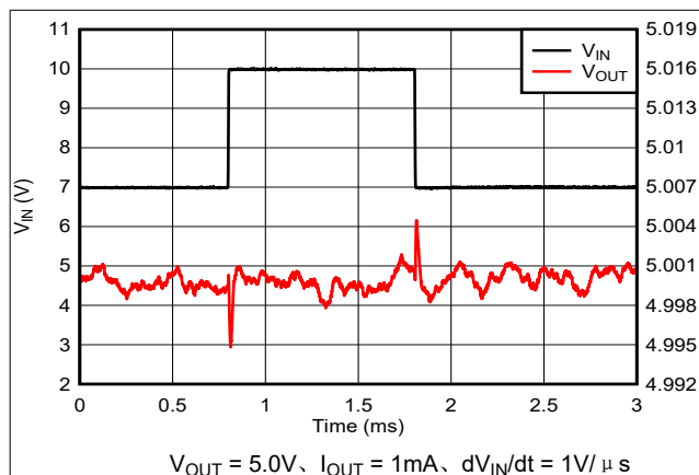
图 7-4. V_{IN} 线路瞬态 (7V 至 10V)
