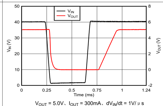
图 5-36. 欠压瞬态 (40V 至 1.7V)
