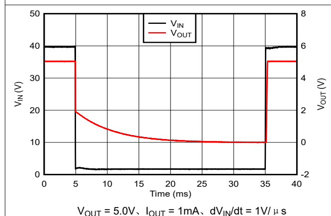
图 5-33. 欠压瞬态 (40V 至 1.7V)
