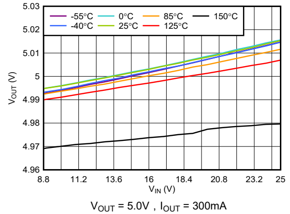
图 5-4. V_{OUT} 与 V_{IN} 间的关系
