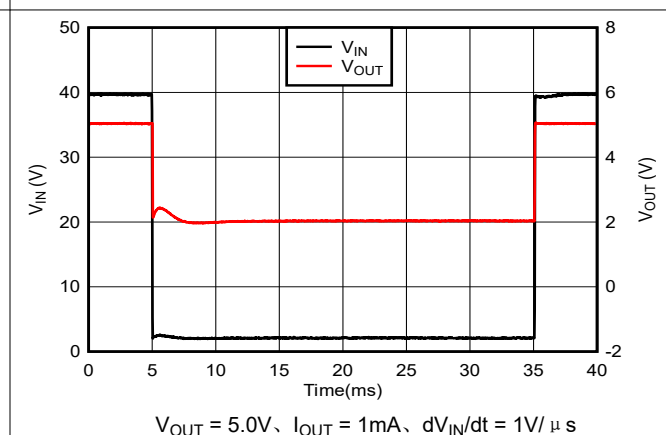
图 5-34. 欠压瞬态 (40V 至 2.1V)
