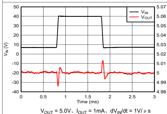
图 7-6. V_{IN} 线路瞬态 (7V 至 40V)
