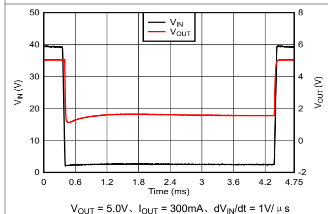
图 5-35. 欠压瞬态 (40V 至 2.5V)
