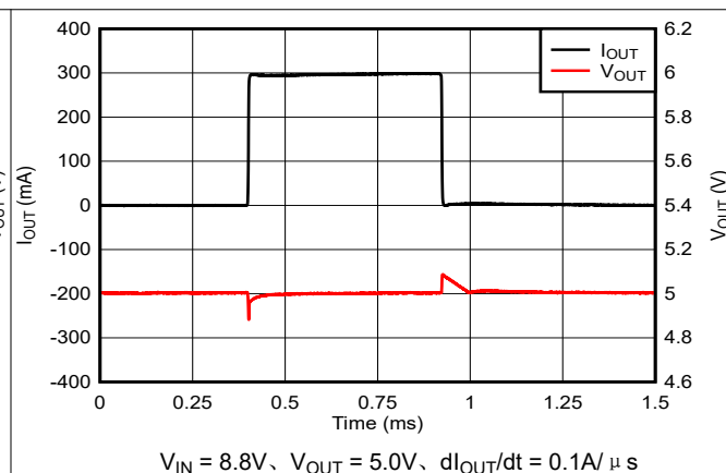
图 5-32. 负载瞬态 (1mA 至 300mA)
