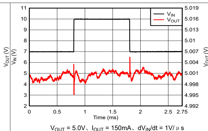
图 7-5. V_{IN} 线路瞬态 (7V 至 10V)
