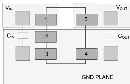
图 7-22. 示例布局
