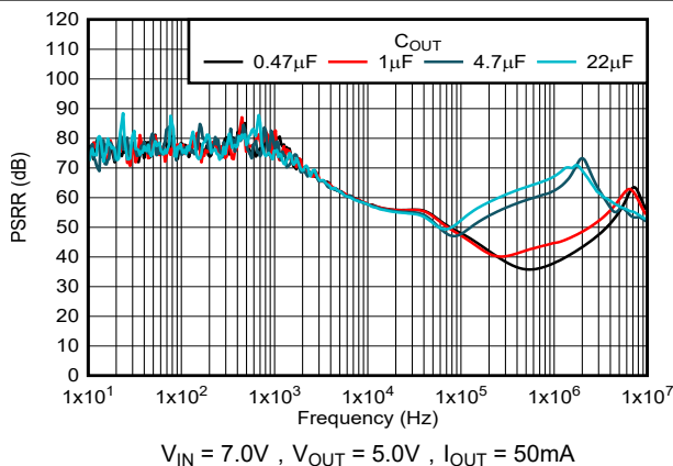
图 5-41. PSRR 与输出电容器间的关系
