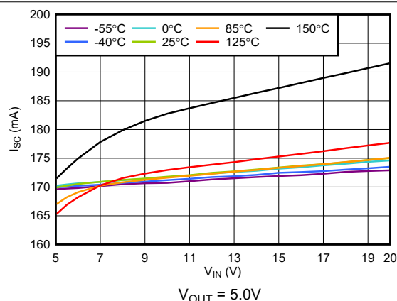
图 5-20. 短路电流限值与 V_{IN} 间的关系
