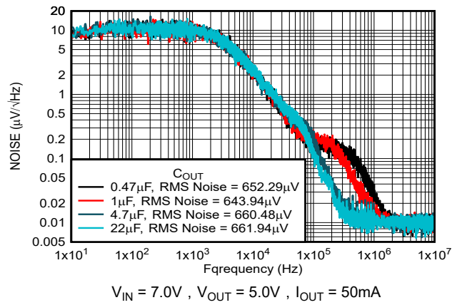
图 5-44. 噪声与输出电容器间的关系
