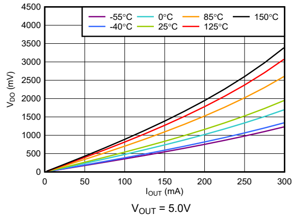
图 5-17. 压降与 I_{OUT} 间的关系
