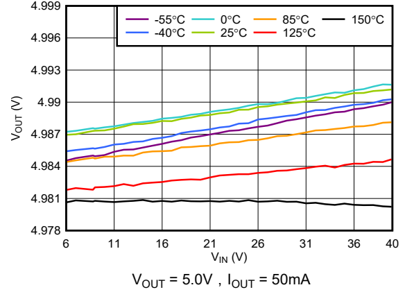
图 5-2. V_{OUT} 与 V_{IN} 间的关系
