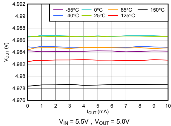
图 5-5. V_{OUT} 与 I_{OUT} 间的关系
