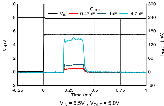
图 5-38. 浪涌电流与输出电容器间的关系
