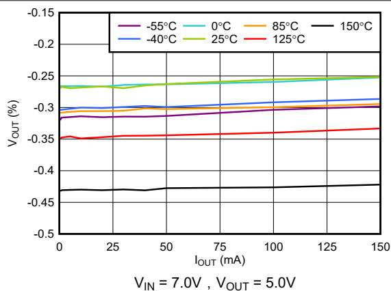
图 5-10. V_{OUT} 精度与 I_{OUT} 间的关系
