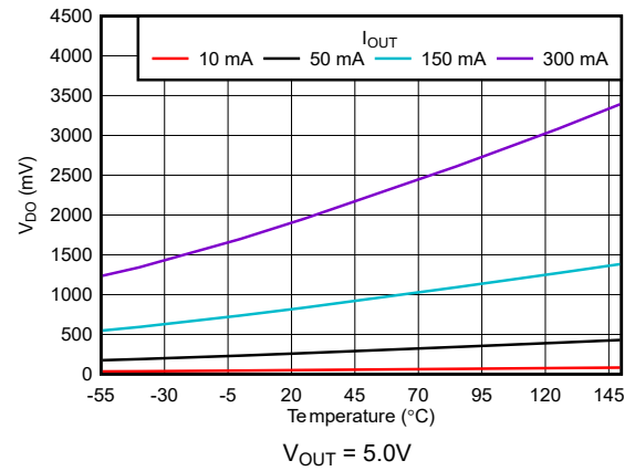
图 5-16. 压降与温度间的关系
