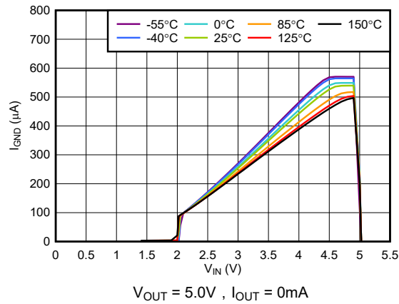
图 5-15. I_{GND} 与 V_{IN} 间的关系 (压降运行)
