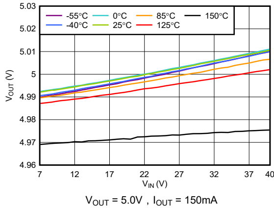
图 5-3. V_{OUT} 与 V_{IN} 间的关系
