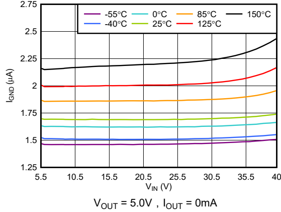
图 5-13. I_{GND} 与 V_{IN} 间的关系
