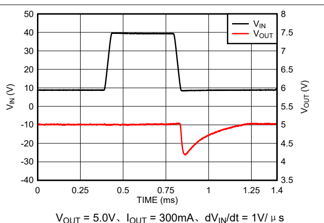
图 7-11. V_{IN} 线路瞬态 (8.8V 至 40V)
