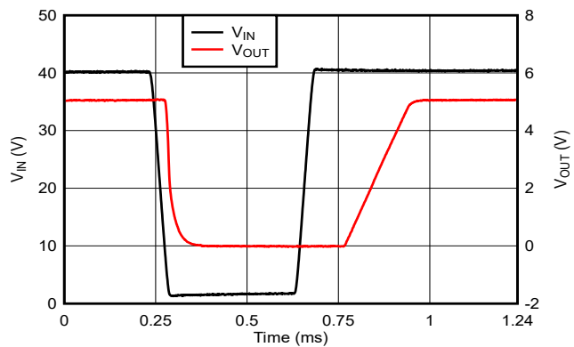
图 7-17. 欠压瞬态 (40V 至 2.1V)
