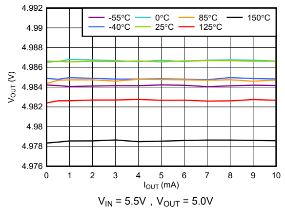
图 5-4. V_{OUT} 与 I_{OUT} 间的关系
