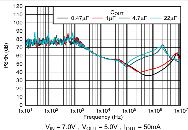
图 5-33. PSRR 与输出电容器间的关系
