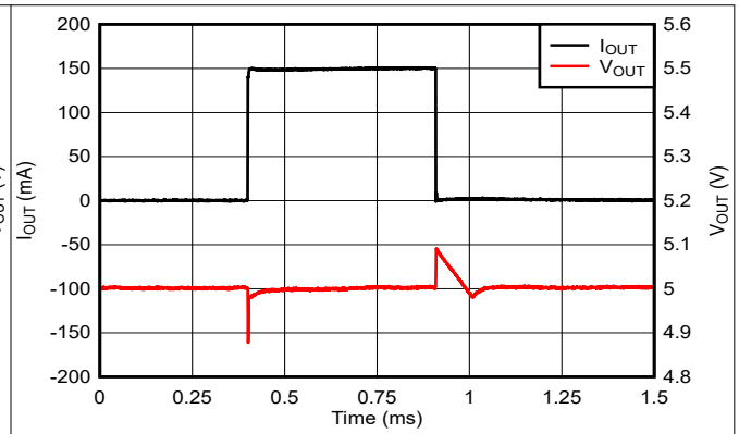
图 5-26. 负载瞬态 (1mA 至 150mA)
