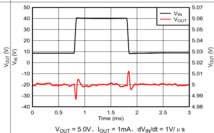
图 7-9. V_{IN} 线路瞬态 (8.8V 至 40V)
