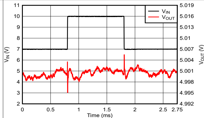
图 5-20. V_{IN} 线路瞬态 (7V 至 10V)
