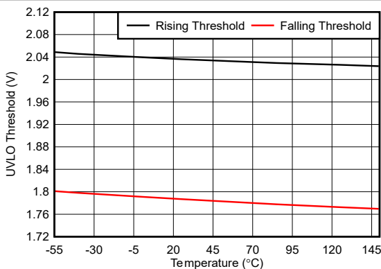
图 5-19. UVLO 阈值与温度间的关系
