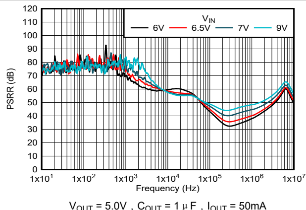
图 5-32. PSRR 与输入电源间的关系
