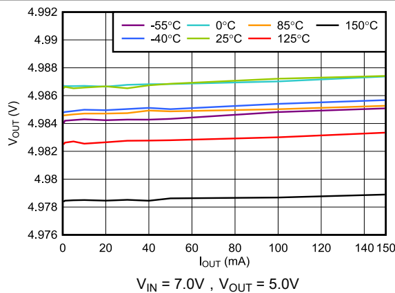
图 5-5. V_{OUT} 与 I_{OUT} 间的关系
