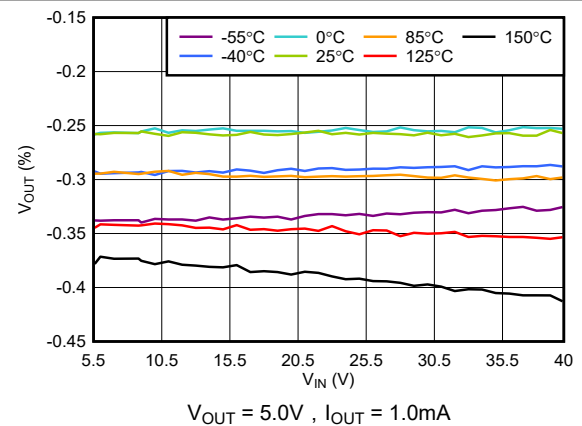
图 5-6. V_{OUT} 精度与 V_{IN} 间的关系
