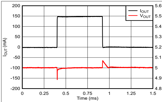
图 5-25. 负载瞬态 (1mA 至 150mA)
