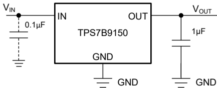
图 7-1. 典型应用电路
