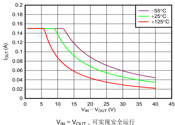
图 7-3. I_{OUT} 与余量 ( V_{IN} - V_{OUT} ) 间的关系
