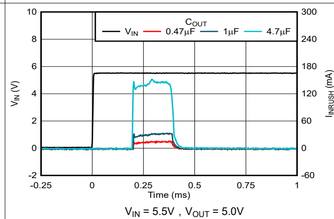
图 5-30. 浪涌电流与输出电容器间的关系
