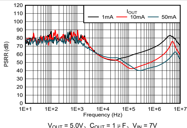
图 5-31. PSRR 与负载电流间的关系
