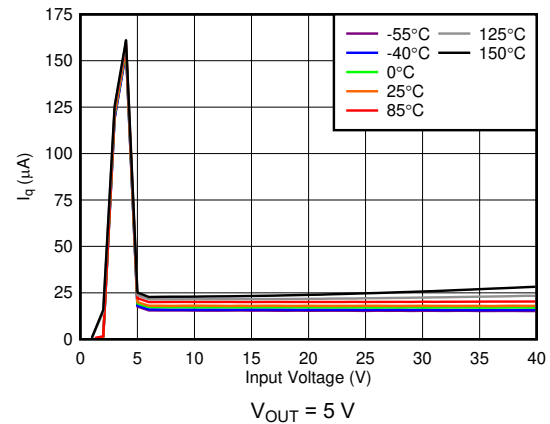
图 6-28. Quiescent Current ( I_Q ) vs V_{IN}
