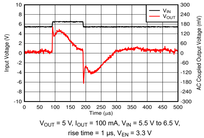
图 6-16. Line Transients
