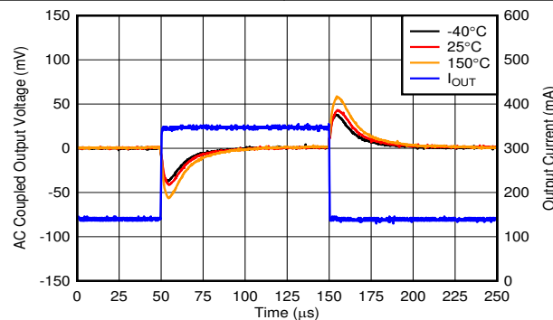
图 8-10. Transient Response
