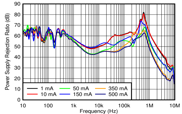
图 8-9. PSRR
