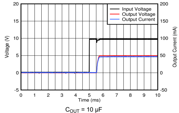
图 6-34. Startup Plot
