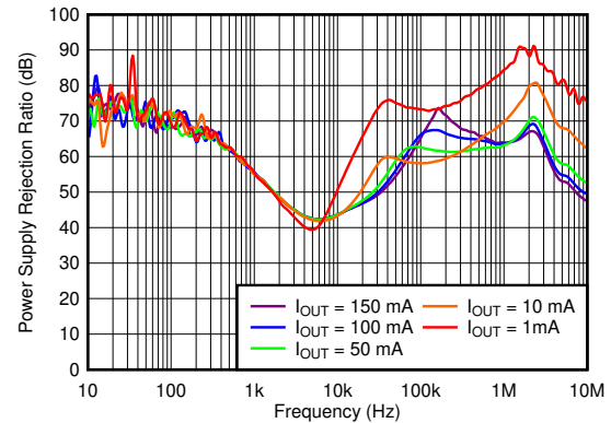
图 8-14. PSRR
