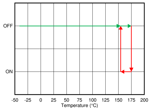
图 6-30. Thermal Shutdown
