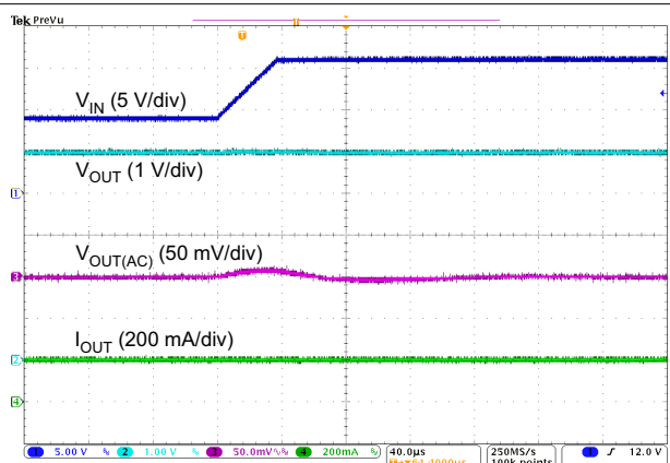
图 5-15. Line Transient
