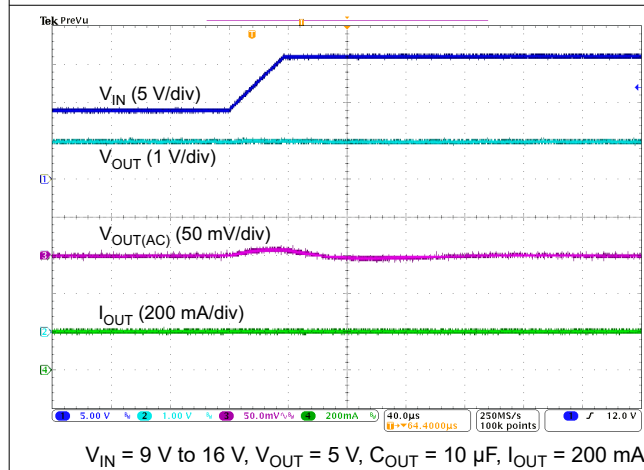
图 6-17. Line Transient
