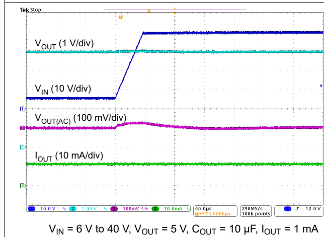
图 6-15. Line Transient
