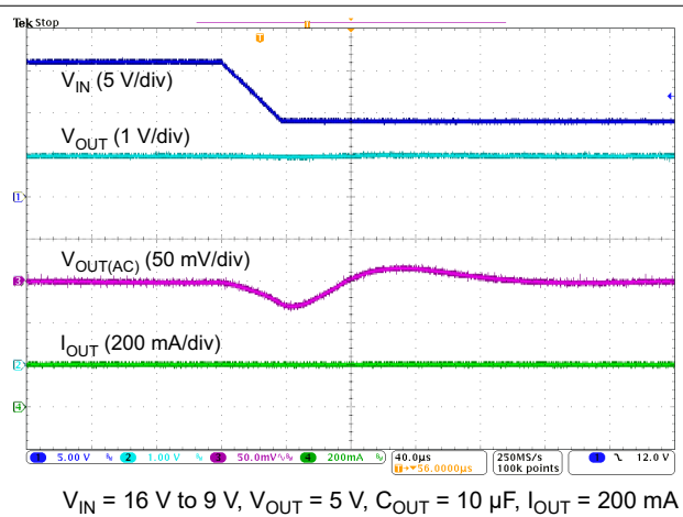
图 6-18. Line Transient
