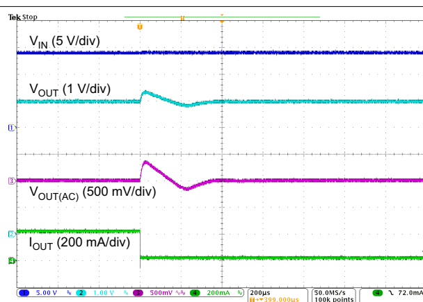
图 5-20. Load Transient
