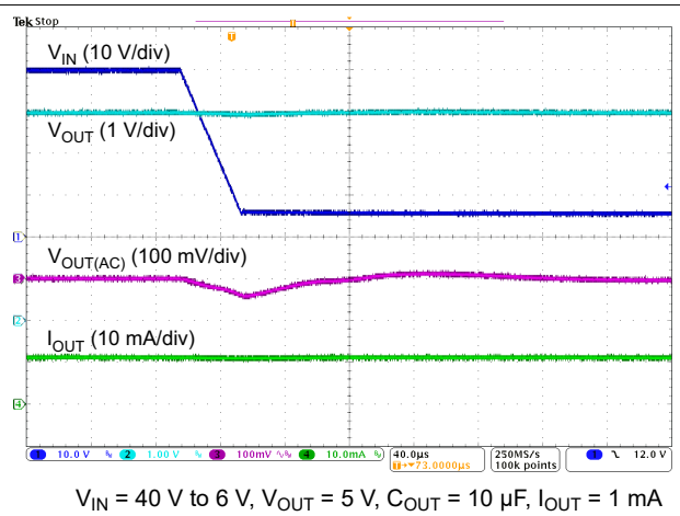
图 6-16. Line Transient
