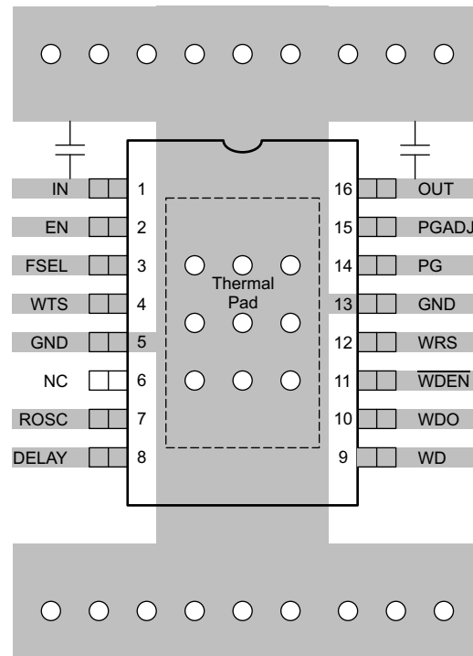
图 8-4. Layout Recommendation
