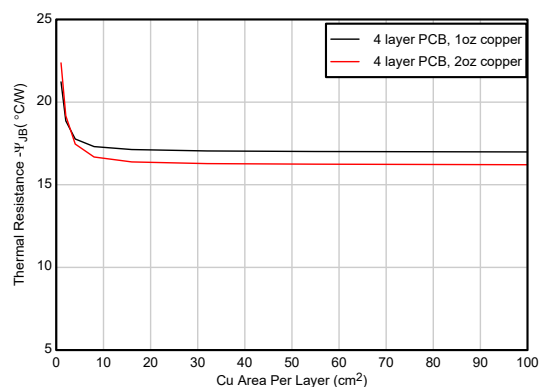
图 7-5. \psi_{JB} 与铜面积间的关系 ( HSOIC-8 封装, 4 层 PCB )
