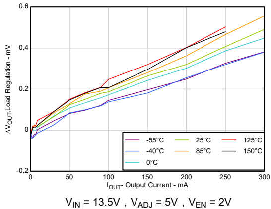
图 5-7. 负载调整率
