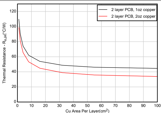
图 7-2. R_{\theta JA} 与铜面积间的关系 ( HSOIC-8 封装, 2 层 PCB )
