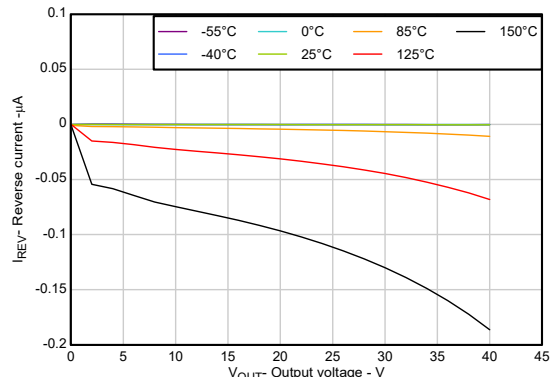
图 5-26. 反向漏电流与输出电压间的关系
