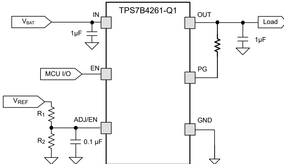
图 6-2. 跟踪器输出电压低于参考电压
