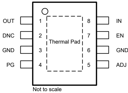
图 4-1. DDA 封装，8 引脚 HSOIC (俯视图)
