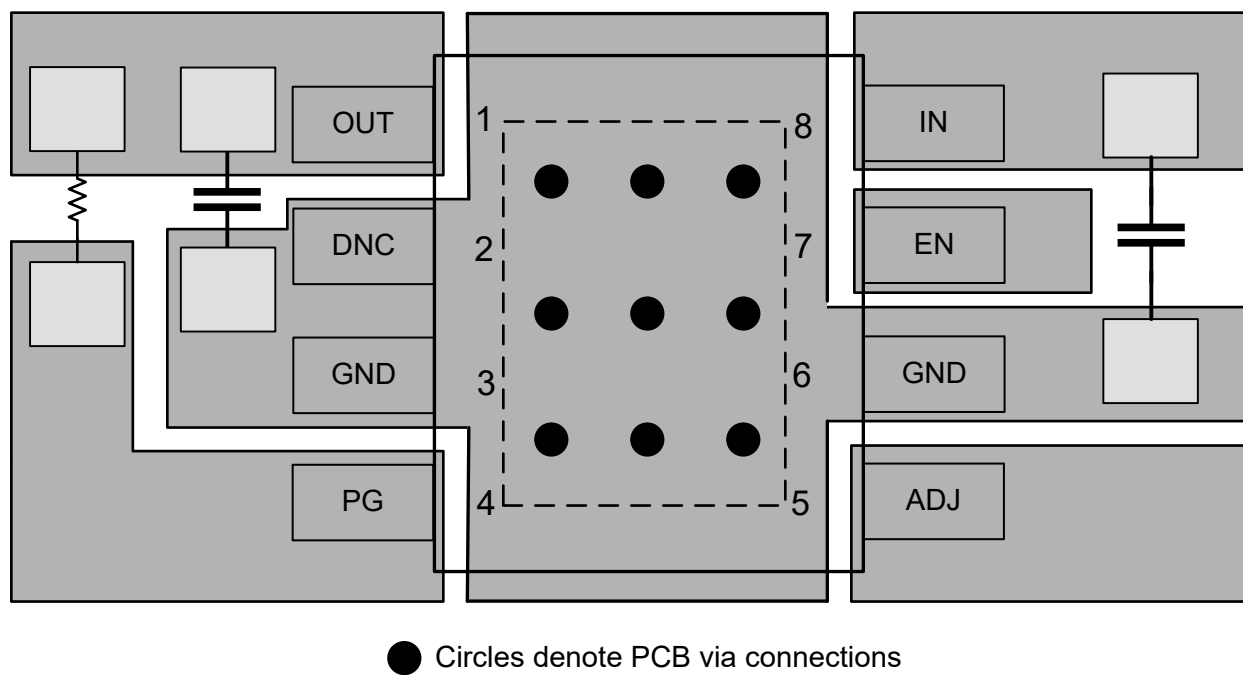
图 7-7. 布局示例
