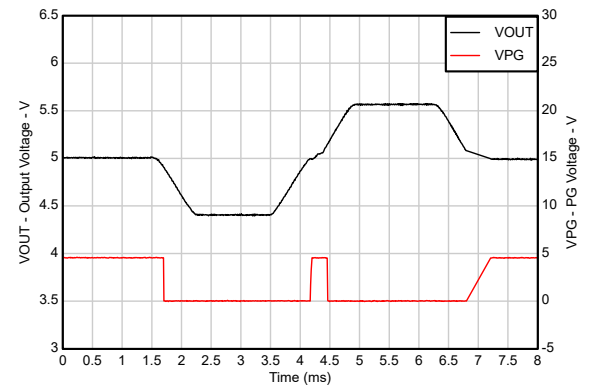
图 5-32. 线路瞬态
