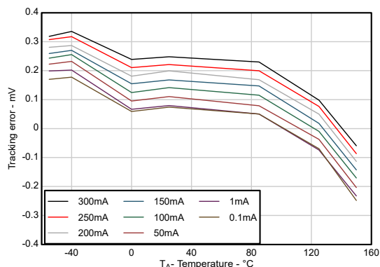
图 5-1. 跟踪误差与环境温度间的关系
