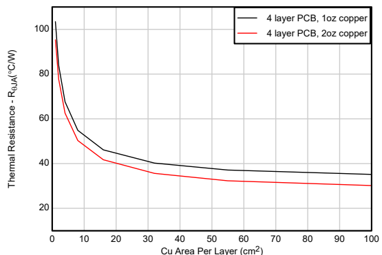
图 7-6. R_{\theta JA} 与铜面积间的关系 ( HSOIC-8 封装, 4 层 PCB )
