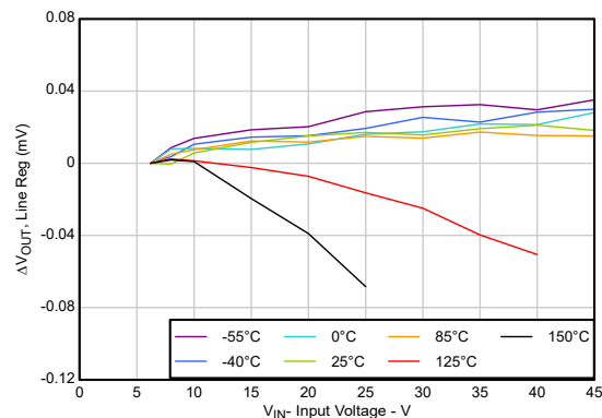
图 5-4. 输出电压与输入电压间的关系
