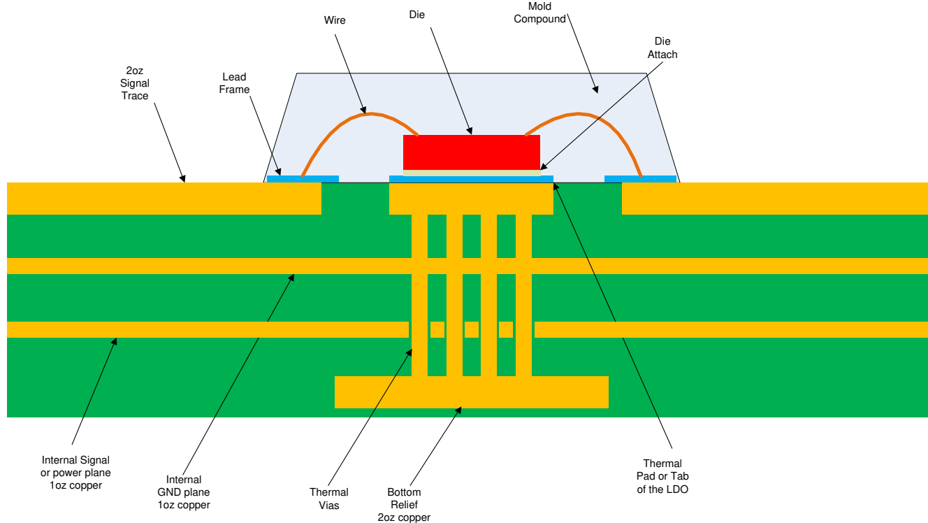
图 7-8. JEDEC 标准 2s2p PCB
