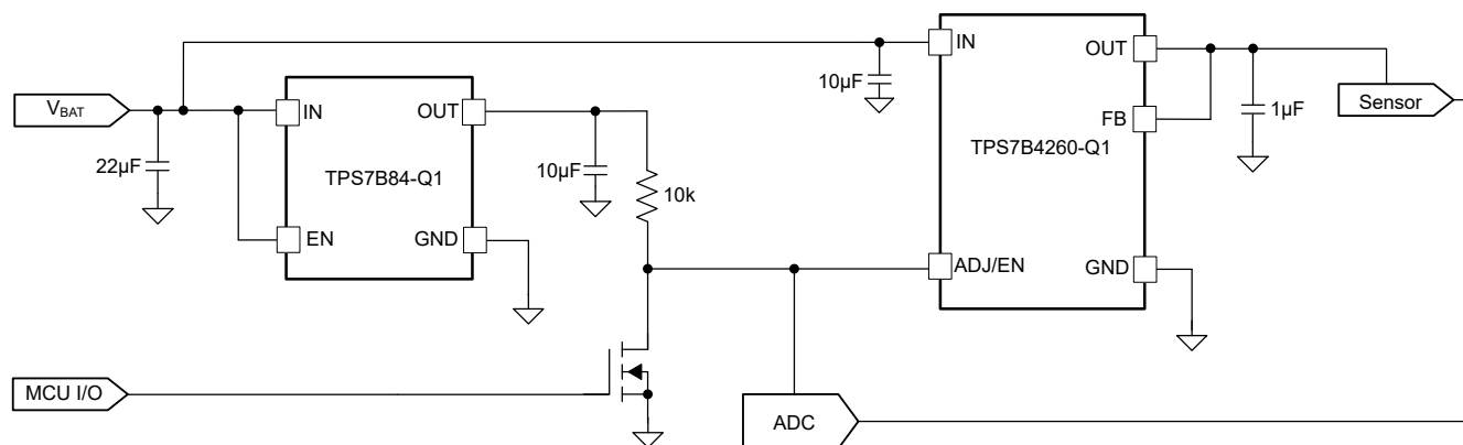
图 6-7. 通过使能电路跟踪 LDO
