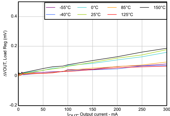
图 5-7. 负载调整率
