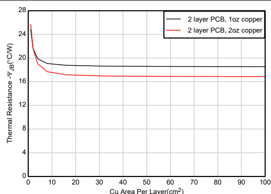
图 7-5. \psi_{JB} 与铜面积间的关系 ( HSOIC-8 封装, 2 层 PCB )
