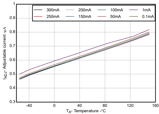
图 5-19. 可调节引脚漏电流与环境温度间的关系
