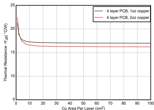
图 7-7. \psi_{JB} 与铜面积间的关系 ( HSOIC-8 封装, 4 层 PCB )
