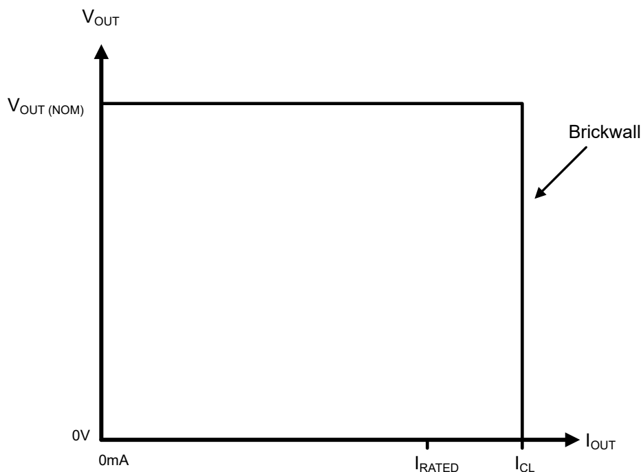
图 6-4. 砖墙电流限制方案
