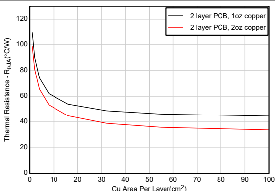
图 7-4. R_{\theta JA} 与铜面积间的关系 ( HSOIC-8 封装, 2 层 PCB )
