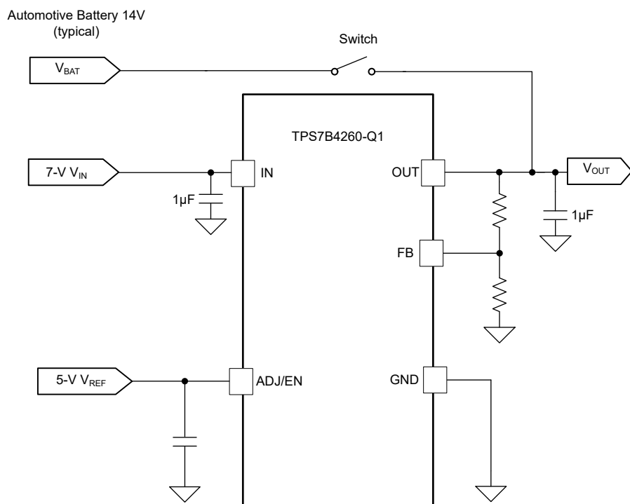
图 6-6. 跟踪器输出电压高于输入电压
