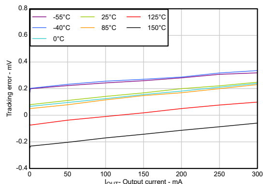
图 5-2. 跟踪误差与输出电流间的关系
