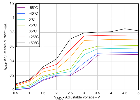
图 5-20. 可调节引脚漏电流与可调节引脚电压间的关系
