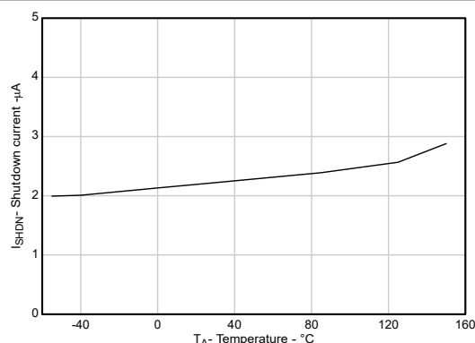
图 5-14. 关断电流与环境温度间的关系
