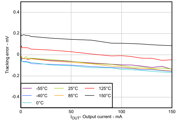
图 5-2. 跟踪误差与输出电流间的关系
