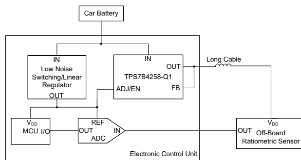
典型应用
