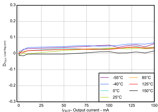
图 5-7. 负载调整率
