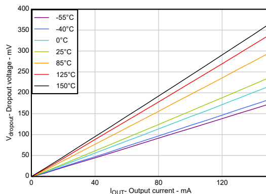
图 5-8. 压降电压与负载电流间的关系
