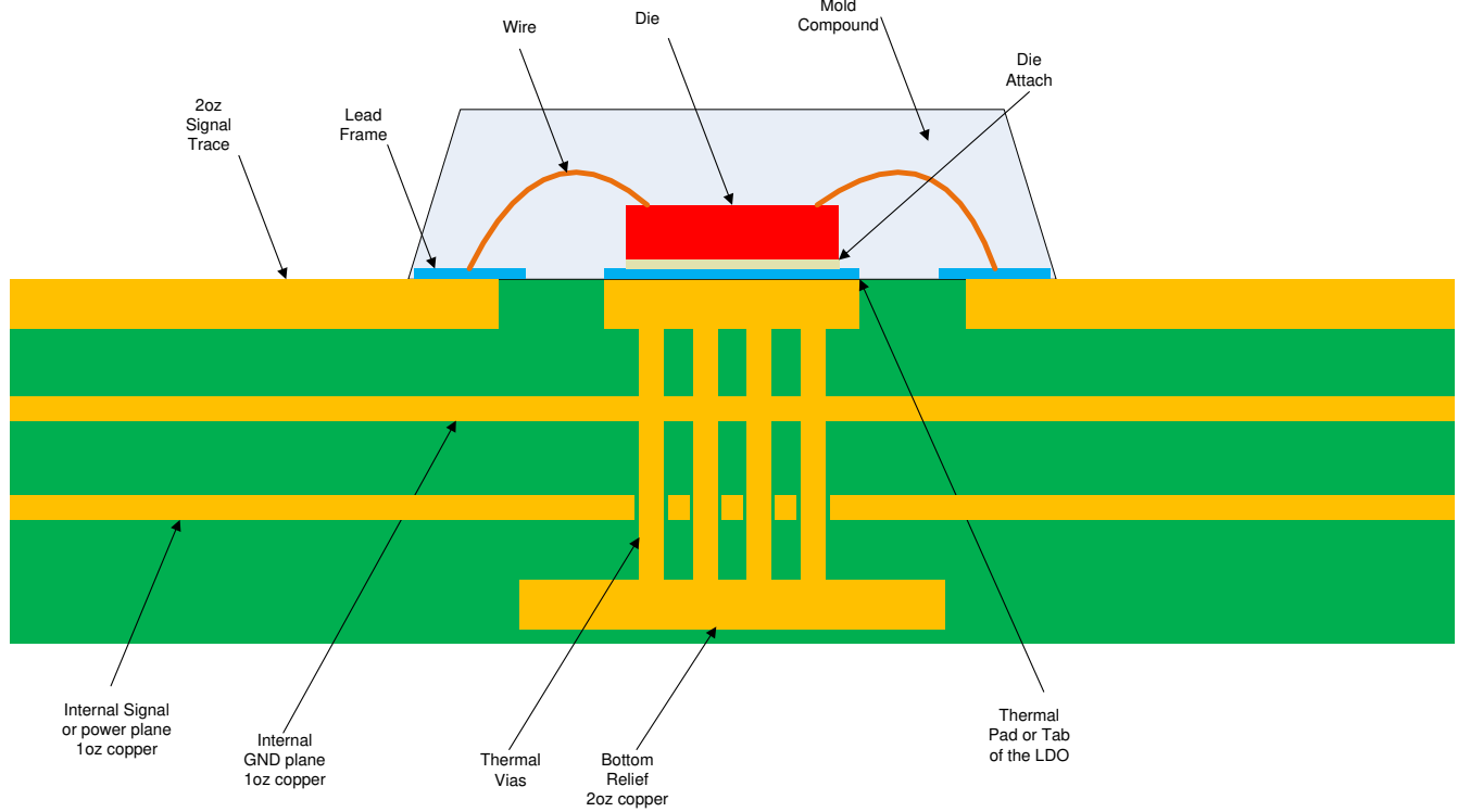
图 7-8. JEDEC 标准 2s2p PCB
