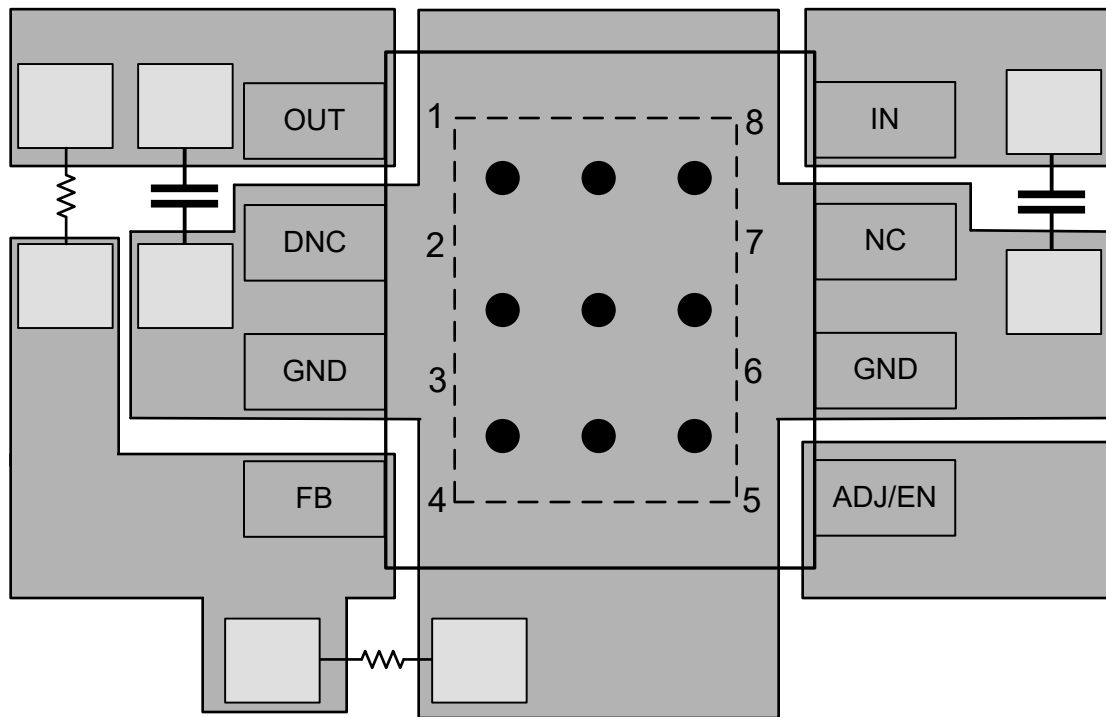
图 7-9. 布局示例
