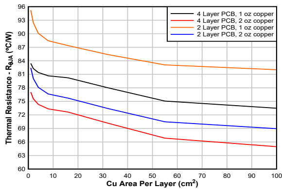
图 7-4. R_{\theta JA} vs Copper Area (SOIC-8 Package)
