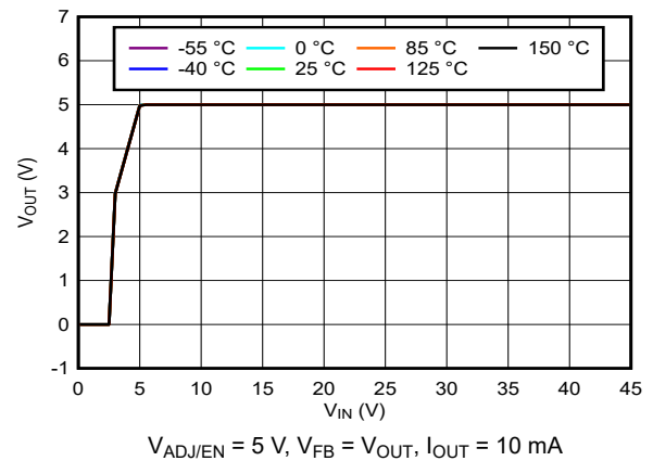
图 5-4. Output Voltage vs Input Voltage
