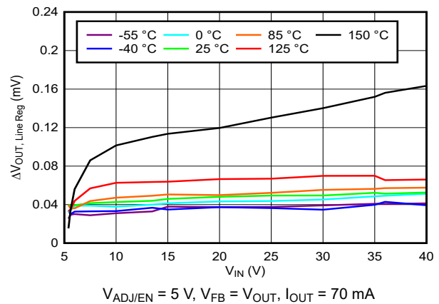
图 5-6. Line Regulation
