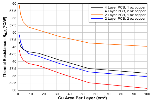
图 7-6. R_{\theta JA} vs Copper Area (HSOIC-8 Package)
