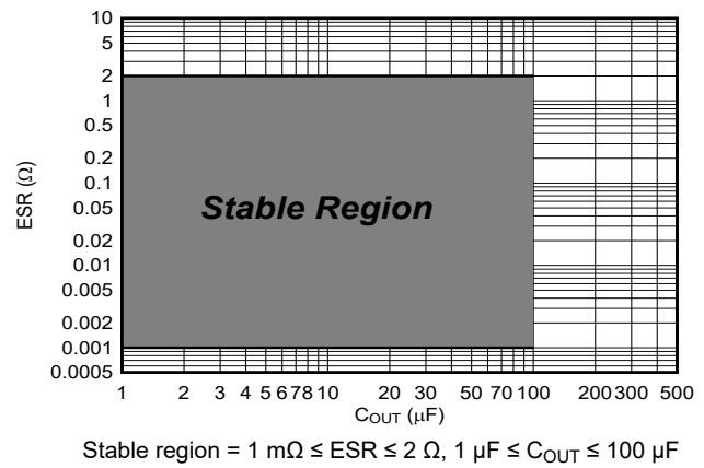
图 5-18. ESR vs Load Capacitance
