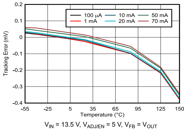
图 5-1. Tracking Error vs Ambient Temperature
