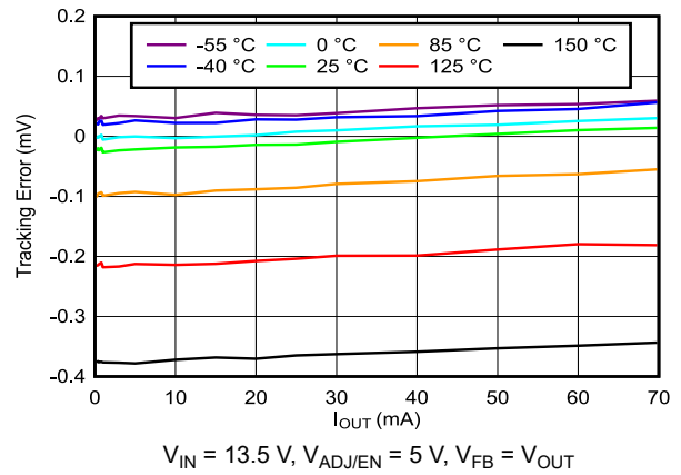
图 5-2. Tracking Error vs Output Current
