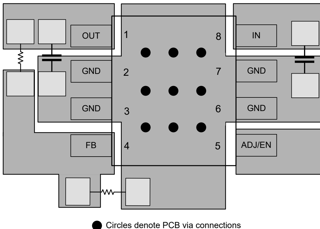
图 7-9. D Package Layout Example
