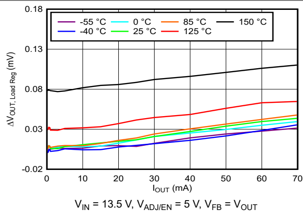
图 5-7. Load Regulation
