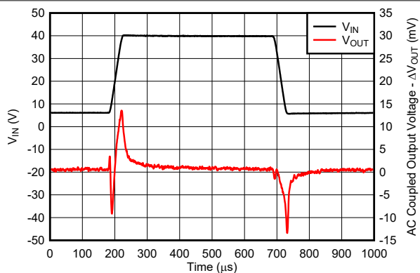
图 5-20. Line Transient
