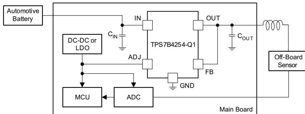
典型应用电路原理图
