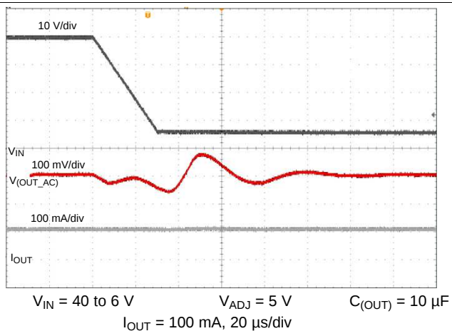
图 17. 40- to 6-V Line Transient
