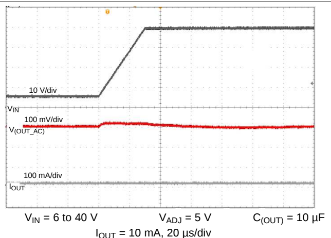
图 18. 6- to 40-V Line Transient
