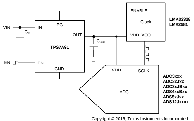
典型应用图
