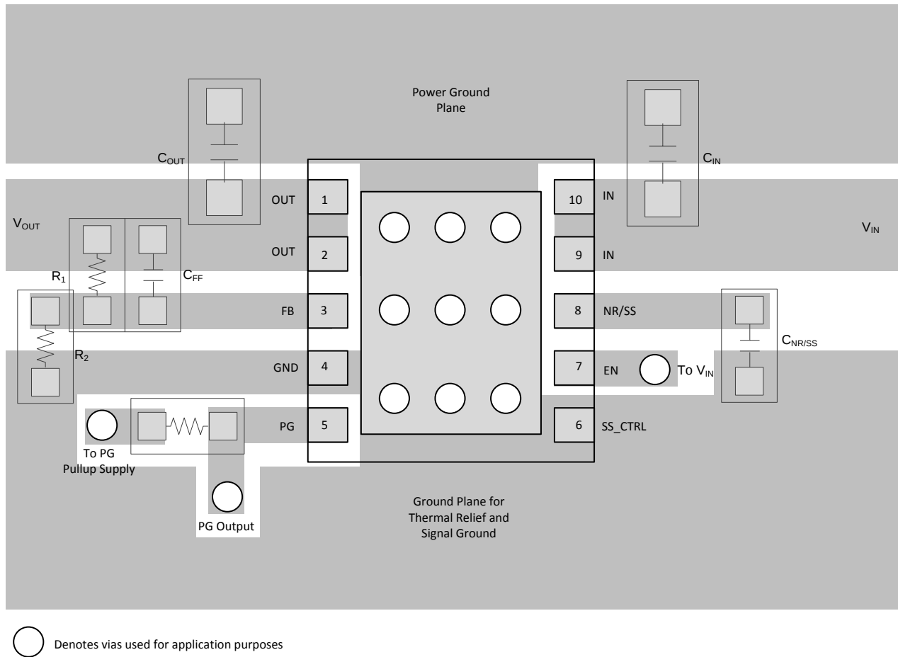
图 42. TPS7A91 Example Layout
