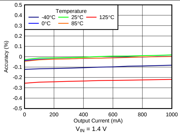
图 16. Load Regulation
