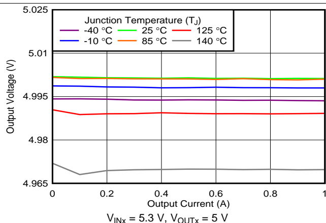
图 29. Load Regulation
