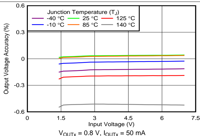
图 26. Line Regulation
