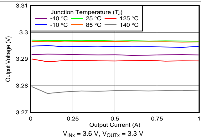
图 27. Load Regulation
