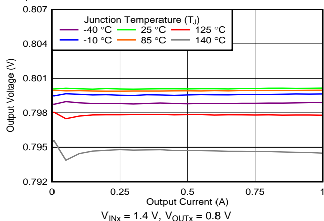
图 25. Load Regulation
