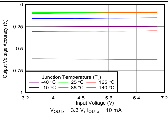
图 28. Line Regulation
