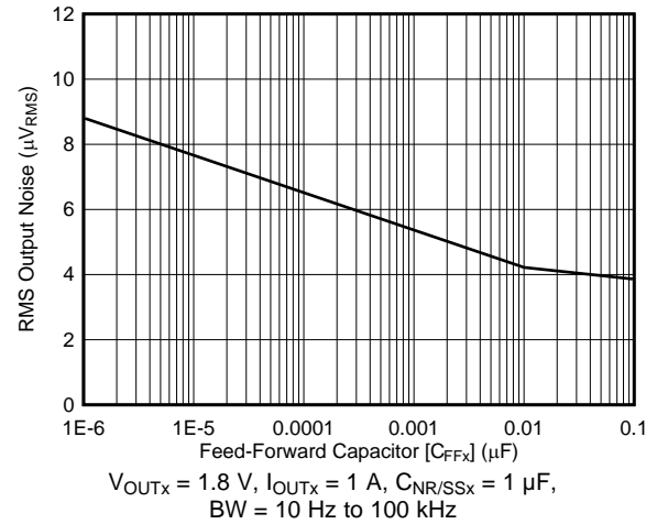
图 14. RMS Output Noise vs C_{\text{FFx}}
