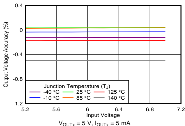
图 30. Line Regulation
