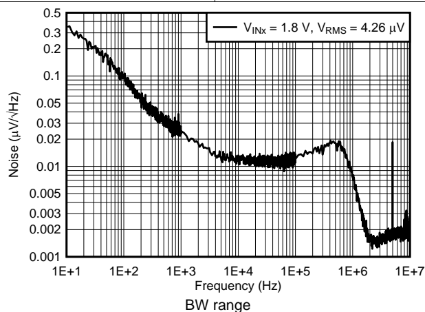
图 58. Output Noise
