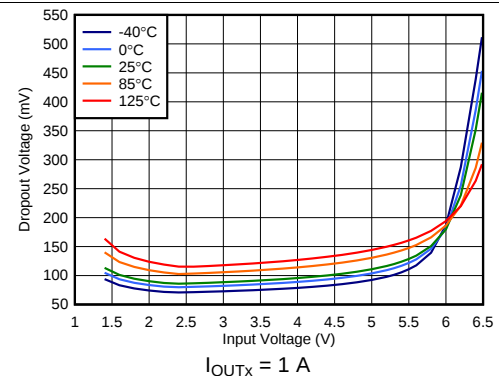
图 24. Dropout Voltage vs Input Voltage
