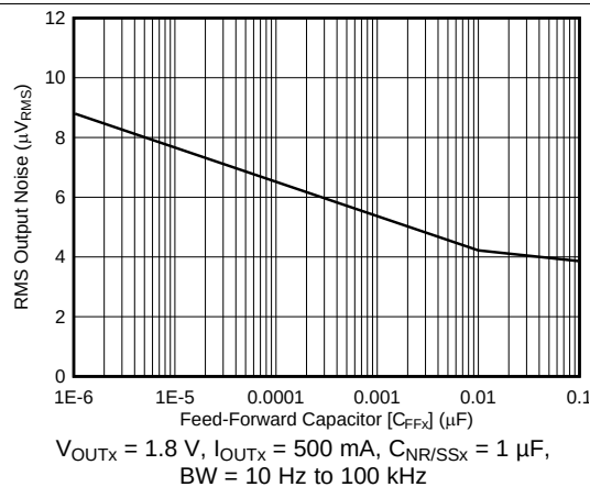
图 15. RMS Output Noise vs C_{\text{FFX}}
