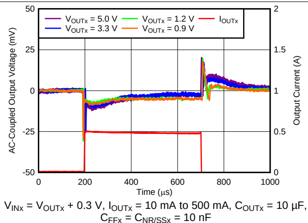
图 16. Load Transient Response vs V_{\text{OUTX}}
