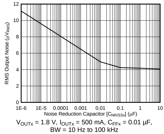
图 14. RMS Output Noise vs C_{\text{NR/SSX}}
