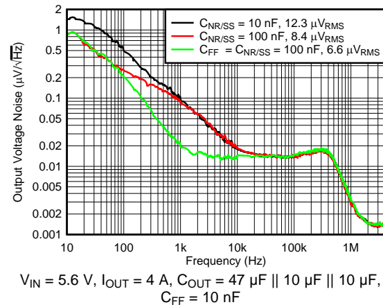
图 16. Output Noise at 5.0-V Output vs C_{NR/SS} and C_{FF}
