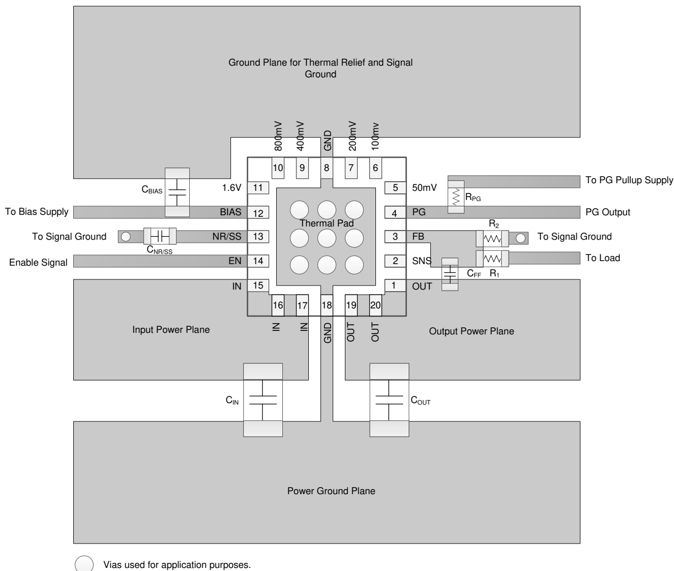
图 10-1. Example Layout
