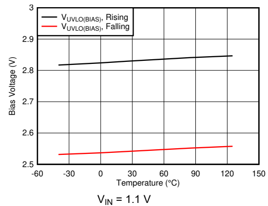
图 6-38. V_{BIAS} UVLO vs Temperature
