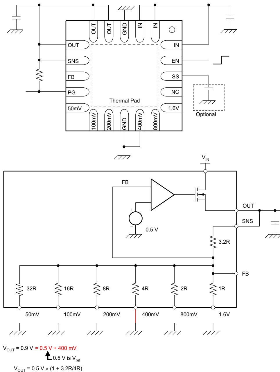
图 6-1. 0.9-V Configuration
