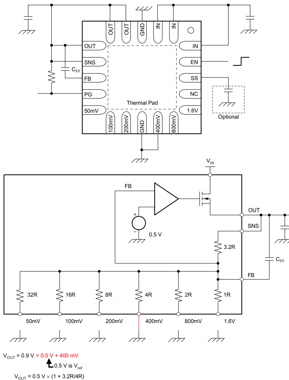
图 6-1. 0.9-V Configuration
