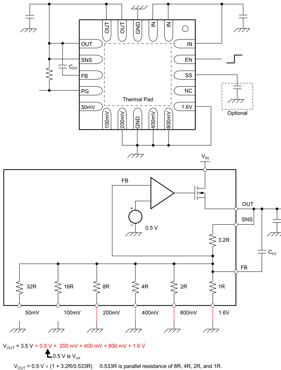
图 6-6. 3.5-V Configuration
