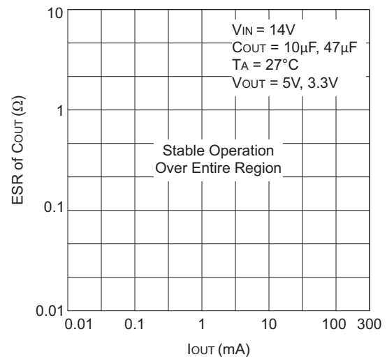
典型稳压器稳定性
