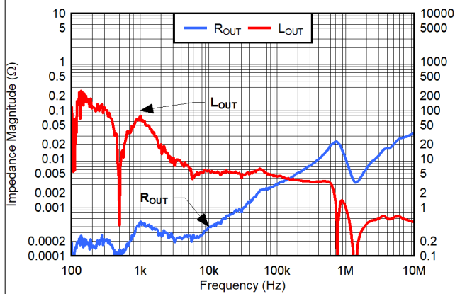
图 8-20. V_{IN} = 0.75\text{ V} , V_{BIAS} = 3\text{ V} , V_{OUT} = 0.5\text{ V} , CP\_EN = 0 , I_{OUT} = 500\text{ mA}
