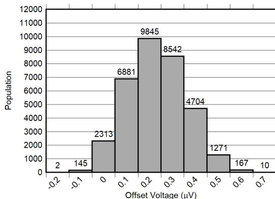
图 6-91. V_{OS} Distribution
