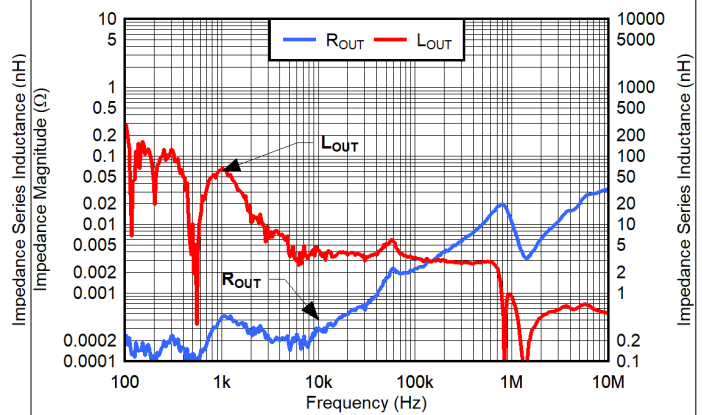
图 8-21. V_{IN} = 0.75\text{ V} , V_{BIAS} = 3\text{ V} , V_{OUT} = 0.5\text{ V} , CP\_EN = 0 , I_{OUT} = 1\text{ A}
