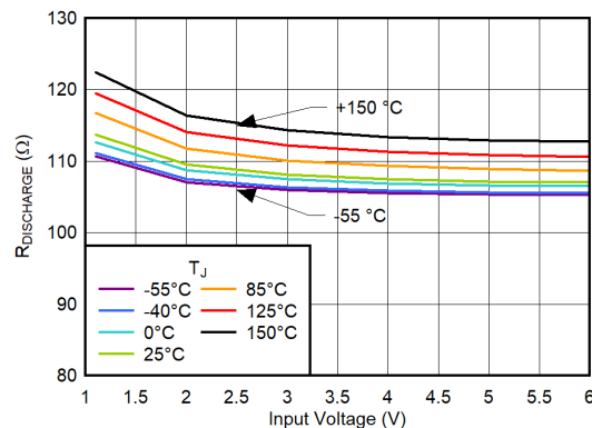
图 6-80. Output Discharge Resistor vs V_{IN}
