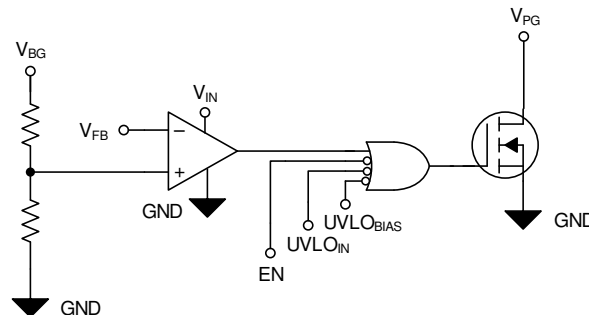
图 6-4. Simplified PG Circuit
