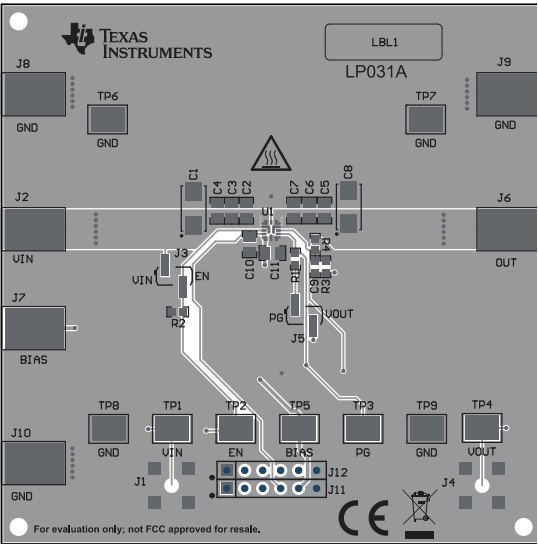
图 7-5. Top Composite View
