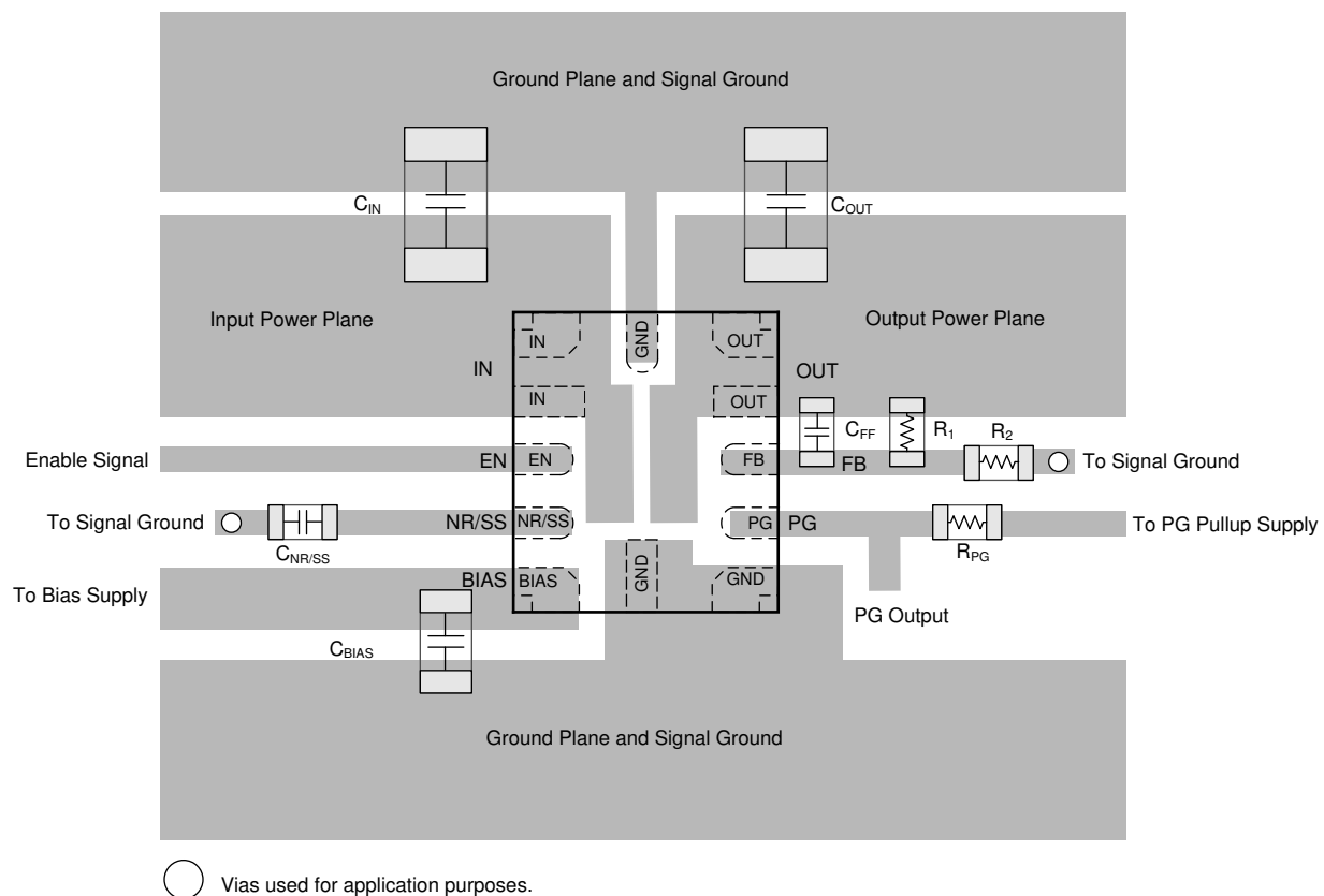
图 7-14. Example Layout
