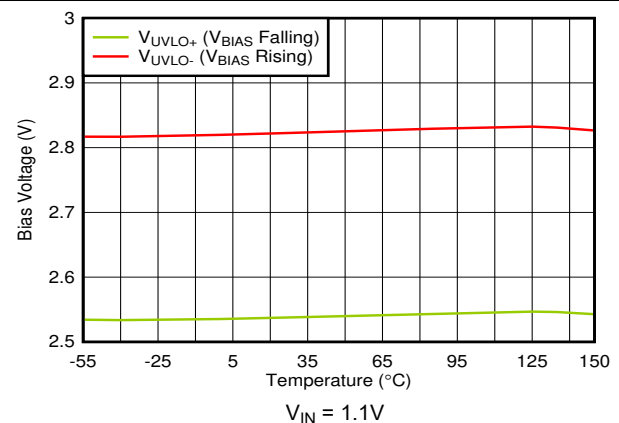
图 5-34. V_{BIAS} UVLO vs Temperature
