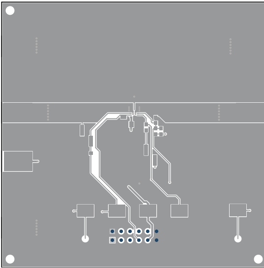
图 7-6. Top Layer Routing
