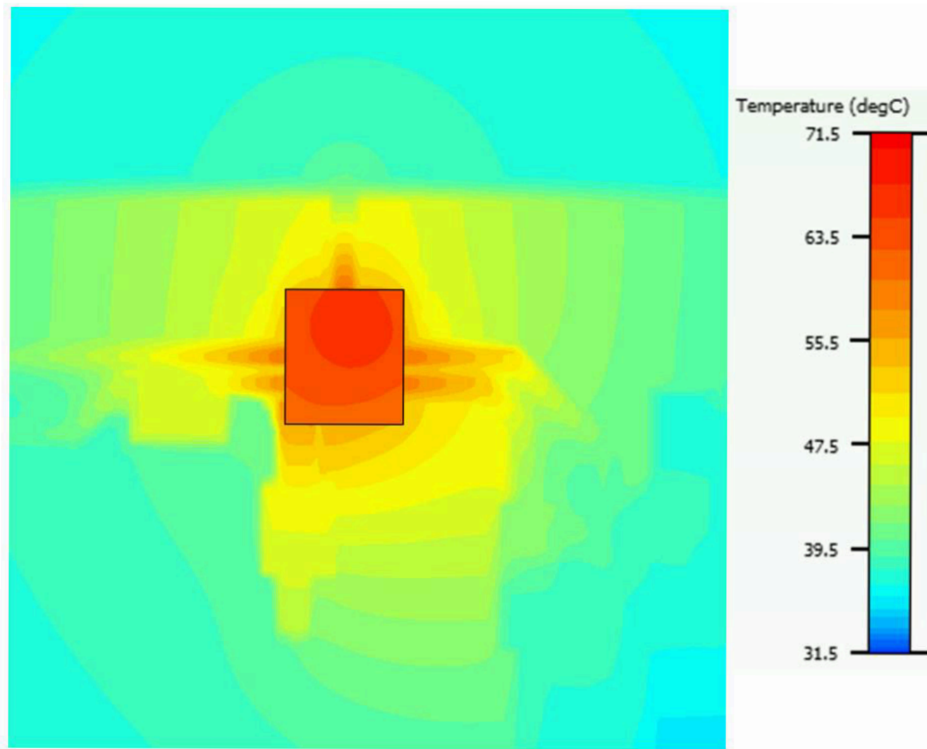
图 7-10. PCB Thermal Gradient
