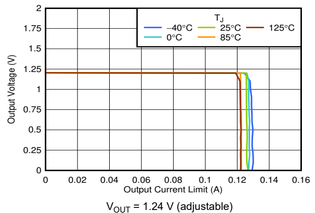
图 6-4. V_{\text{OUT}} vs I_{\text{CL}}(\text{OUT})
