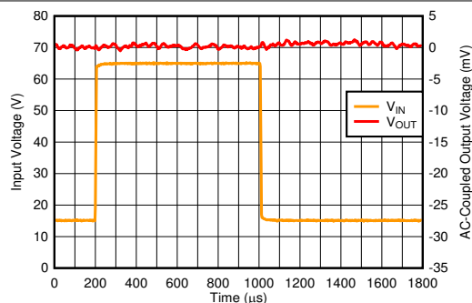
图 6-20. Line Transient
