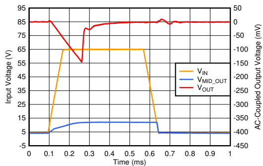
图 6-21. Line Transient
