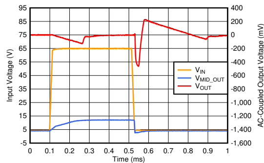
图 6-22. Line Transient
