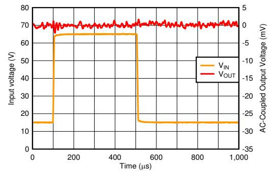
图 6-14. Line Transient
