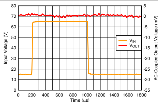
图 6-20. Line Transient
