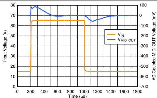
图 6-19. Line Transient
