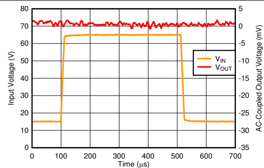
图 6-16. Line Transient
