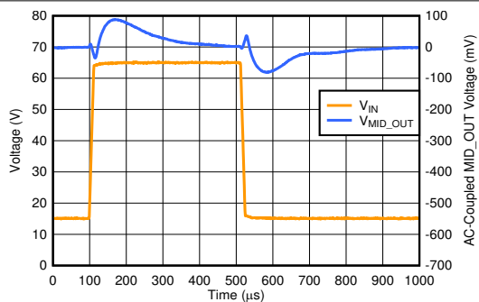
图 6-15. Line Transient
