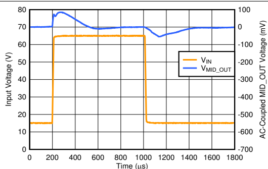
图 6-19. Line Transient
