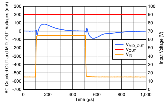
图 6-14. Line Transient
