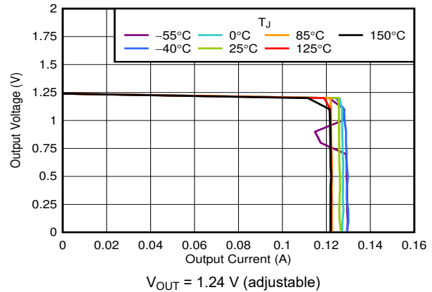
图 6-4. V_{\text{OUT}} vs I_{\text{CL(OUT)}}
