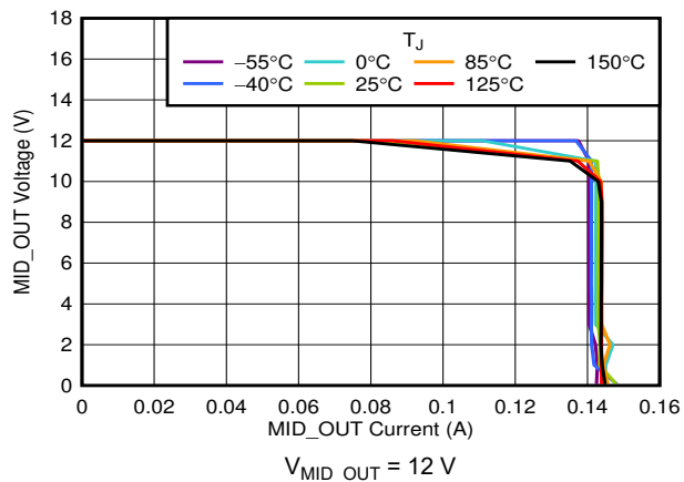
图 6-5. V_{\text{MID\_OUT}} vs I_{\text{MID\_OUT}}
