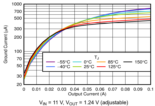
图 6-6. I_{\text{GND}} vs I_{\text{OUT}} ( V_{\text{MID\_OUT}} in Dropout)
