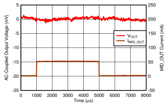
图 6-27. Load Transient (MID_OUT)
