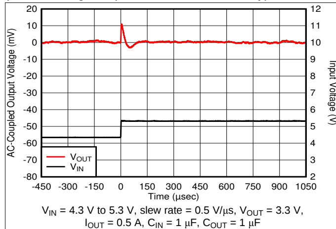
图 31. Line Transient
