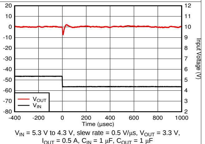
图 30. Line Transient
