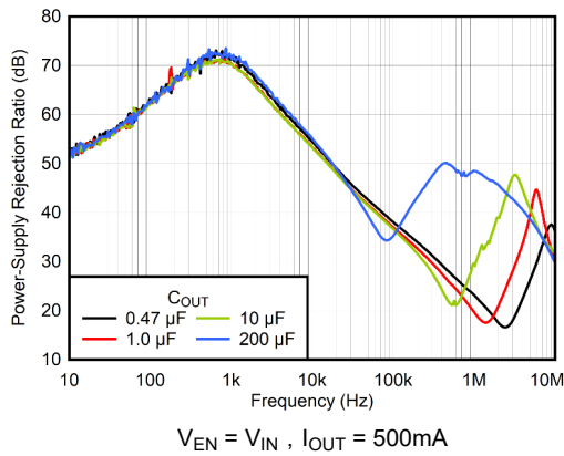
图 5-37. PSRR 与频率和 C_{OUT} 间的关系
