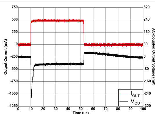
图 5-32. 从 0mA 至 500mA 的负载瞬态
