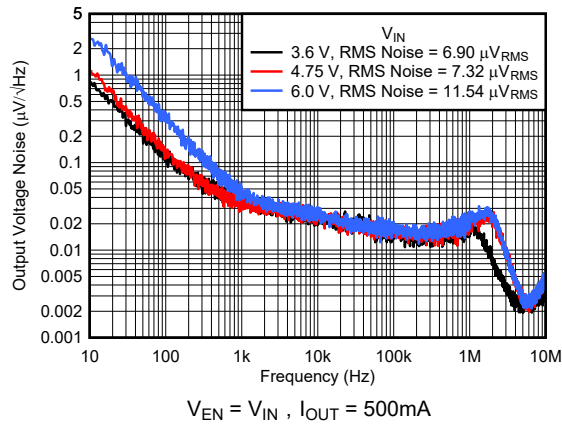
图 5-39. 噪声与频率和 V_{IN} 间的关系
