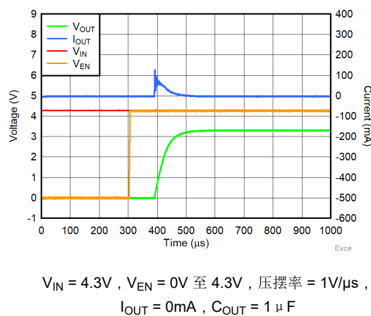
图 5-24. 启动浪涌电流
