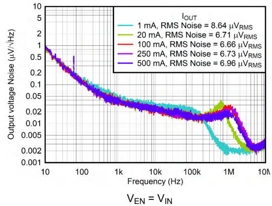
图 5-40. 噪声与频率和 I_{OUT} 间的关系
