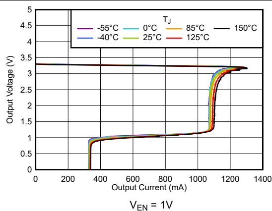
图 5-14. 折返电流限制
