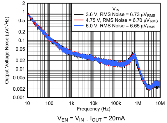
图 5-38. 噪声与频率和 V_{IN} 间的关系
