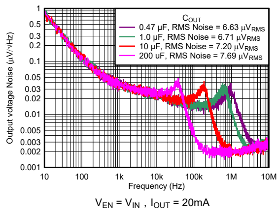
图 5-41. 噪声与频率和 C_{OUT} 间的关系
