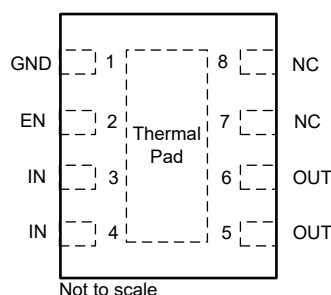
图 4-3. DSG 封装 (DSG0008A)，8 引脚固定 WSON C 版本 (顶视图)
