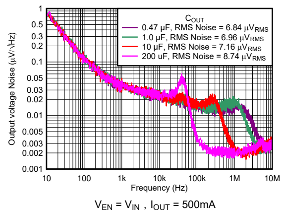
图 5-42. 噪声与频率和 C_{OUT} 间的关系
