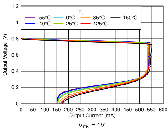
图 5-9. 电流限制
