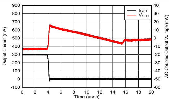
图 5-20. 负载瞬态
