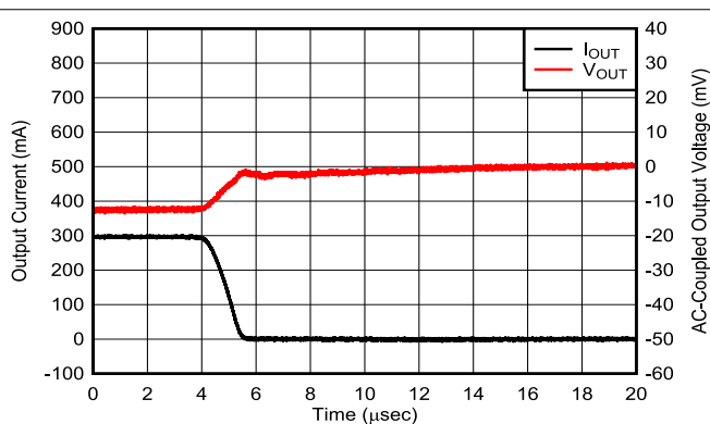
图 5-20. 负载瞬态
