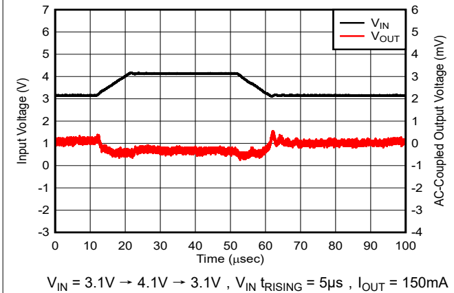
图 5-27. 线路瞬态
