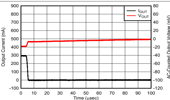
图 5-22. 负载瞬态
