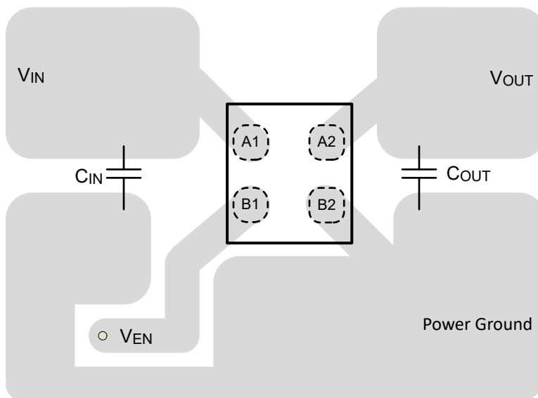
图 7-6. YCK 封装 (DSBGA) 典型布局
