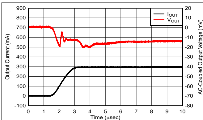
图 5-19. 负载瞬态
