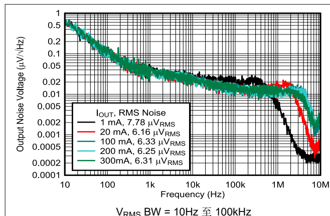
图 5-31. 噪声与频率和 I_{OUT} 间的关系
