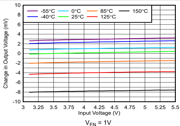
图 5-1. 线路调整率
