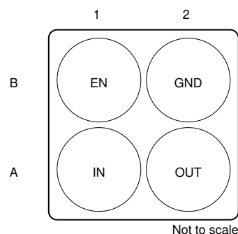
图 4-2. YCK 封装， 4 引脚 DSBGA（底视图）
