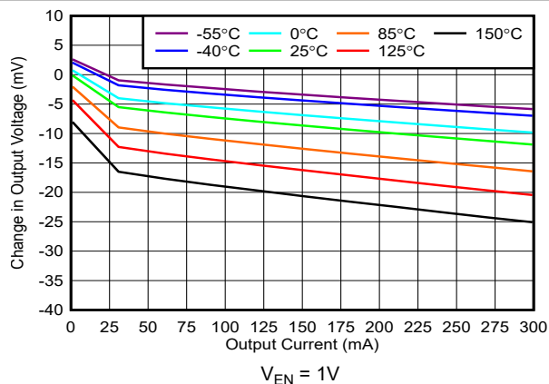
图 5-2. 负载调整率
