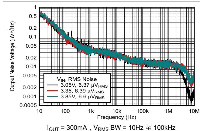
图 5-33. 噪声与频率和 V_{IN} 间的关系
