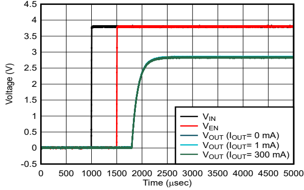
图 5-37. 启动
