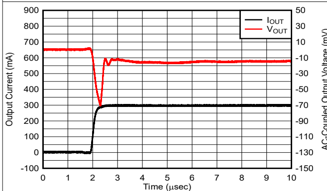
图 5-19. 负载瞬态
