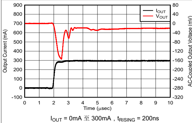
图 5-25. 负载瞬态
