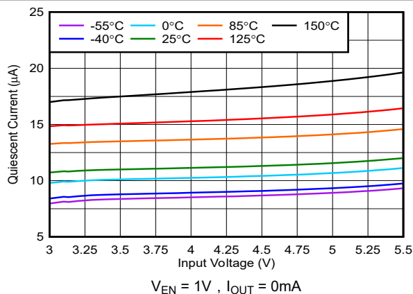
图 5-4. I_{GND} 与 V_{IN} 间的关系
