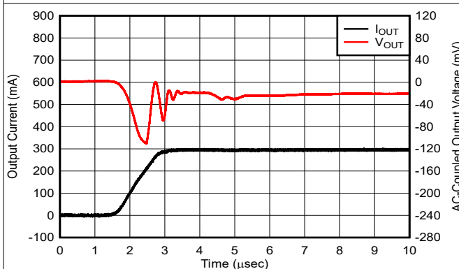
图 5-21. 负载瞬态
