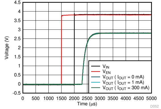
图 5-38. 启动
