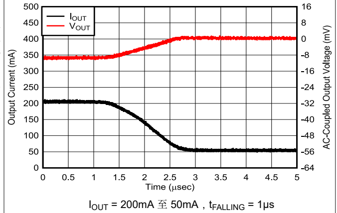
图 5-16. 负载瞬态
