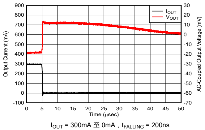
图 5-26. 负载瞬态
