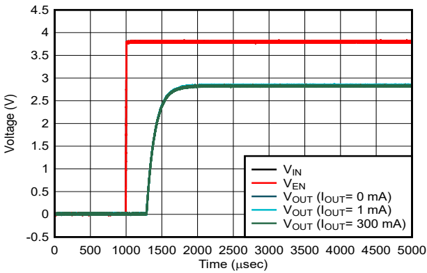
图 7-5. 启动
