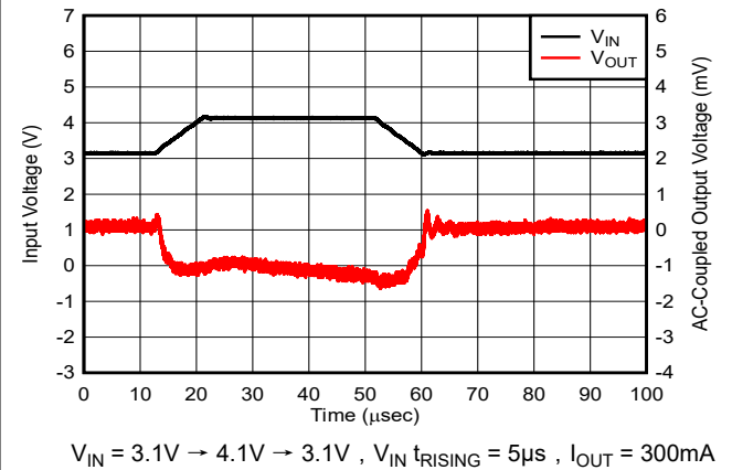
图 5-28. 线路瞬态
