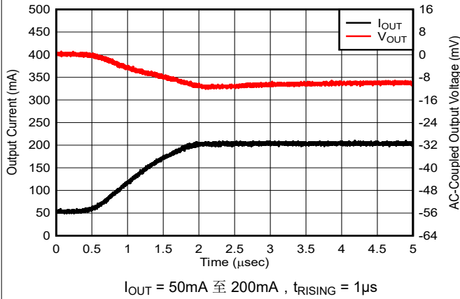
图 5-15. 负载瞬态
