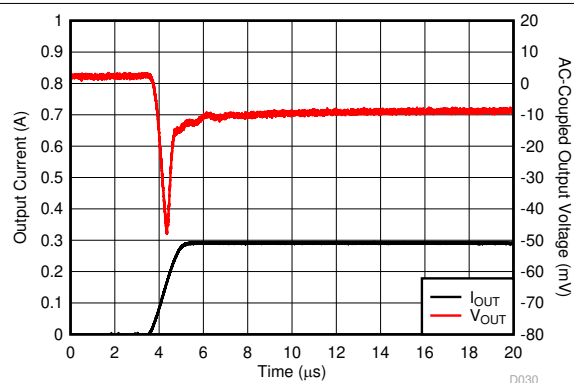
图 5-51. Load Transient
