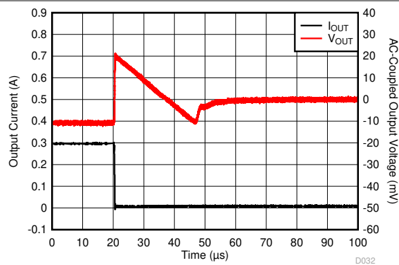
图 5-52. Load Transient
